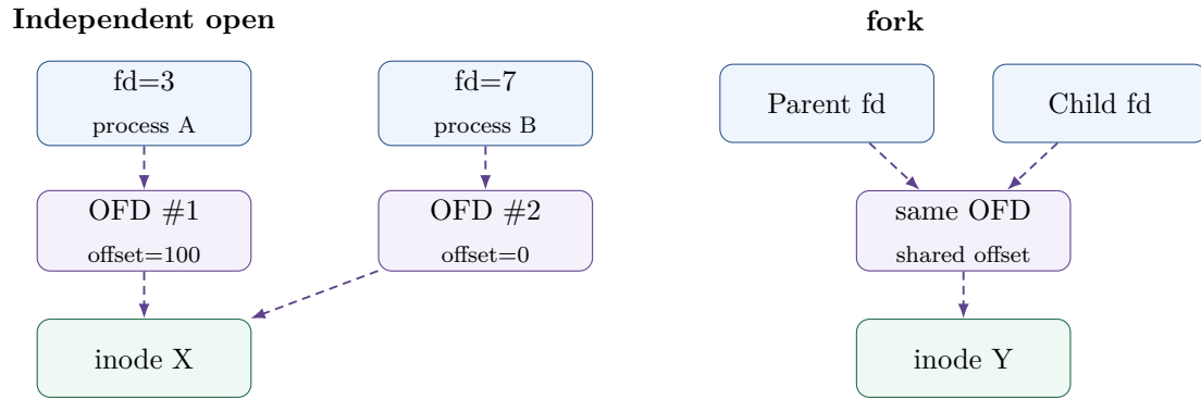
图 3: 独立 open 产生独立 OFD; fork 后对应 fd 引用同一 OFD, 因此共享 file offset。
