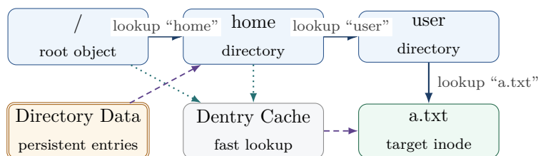
图 1：路径解析：先沿目录逐级推进，dcache 是可选 fast path，而不是磁盘目录项本身。
