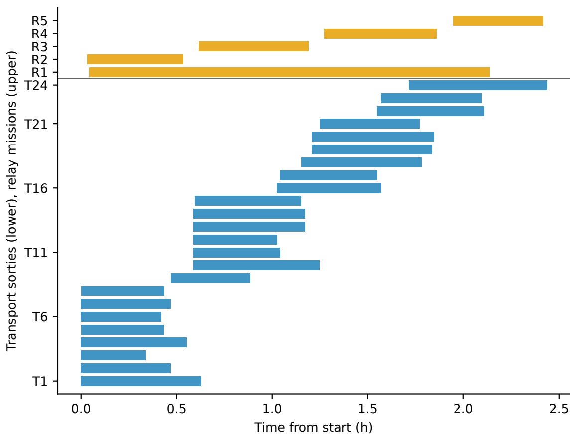
图 2.6 第三问运输与中继任务的联合时间安排; T1-T24 为运输架次, R1-R5 为中继架次
