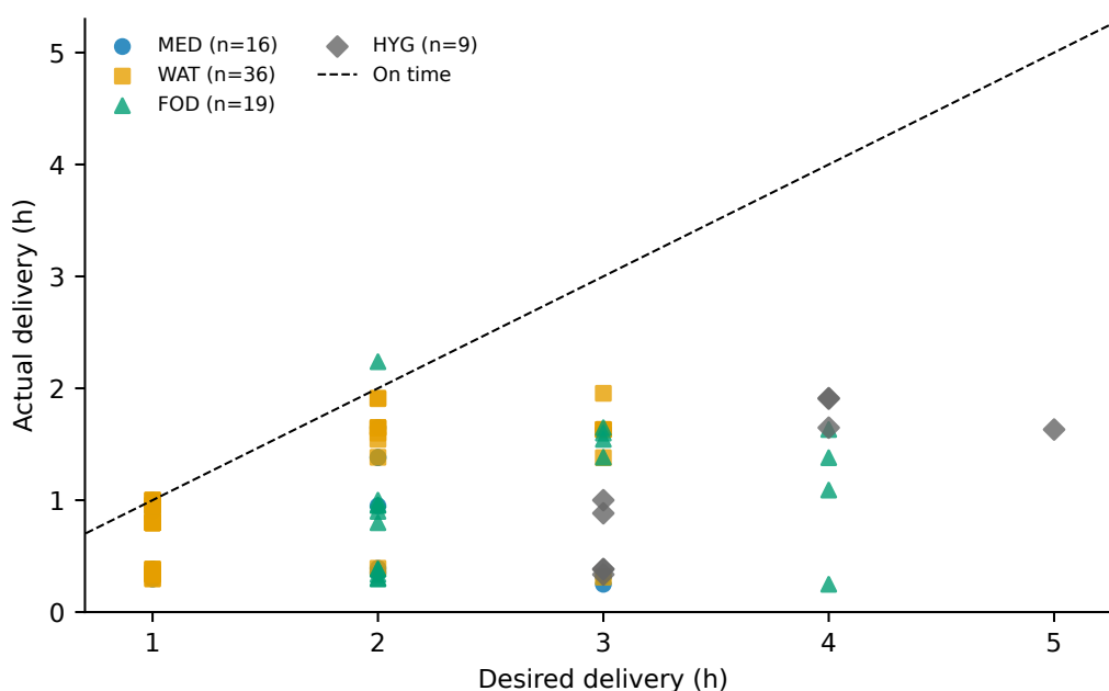
图 2.7 问题三 80 箱的实际与期望交付时刻；虚线表示两者相等
