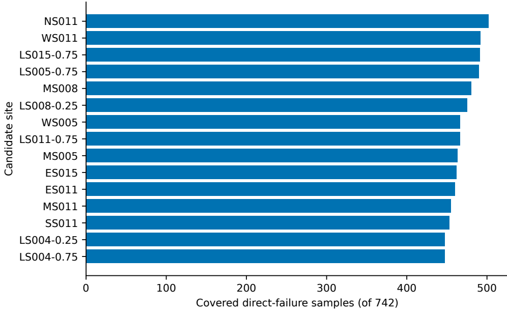
图 5.6 候选中继点对初始运输轨迹直连失效采样点的覆盖数量；每个候选点独立统计
