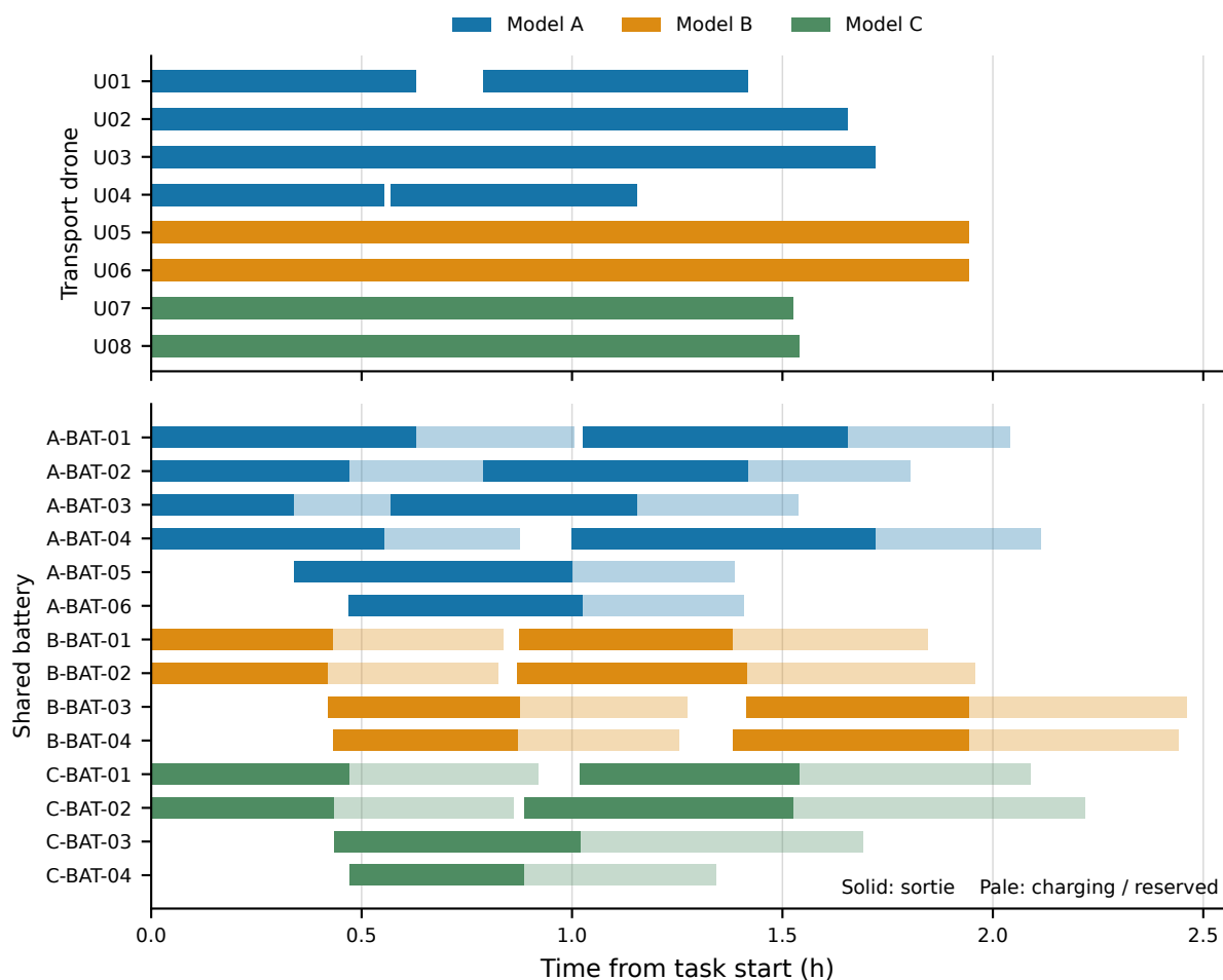
图 4.3 问题二正式方案的运输机与共享电池占用时间轴；浅色部分为返航后的电池充电和保守预留区间
