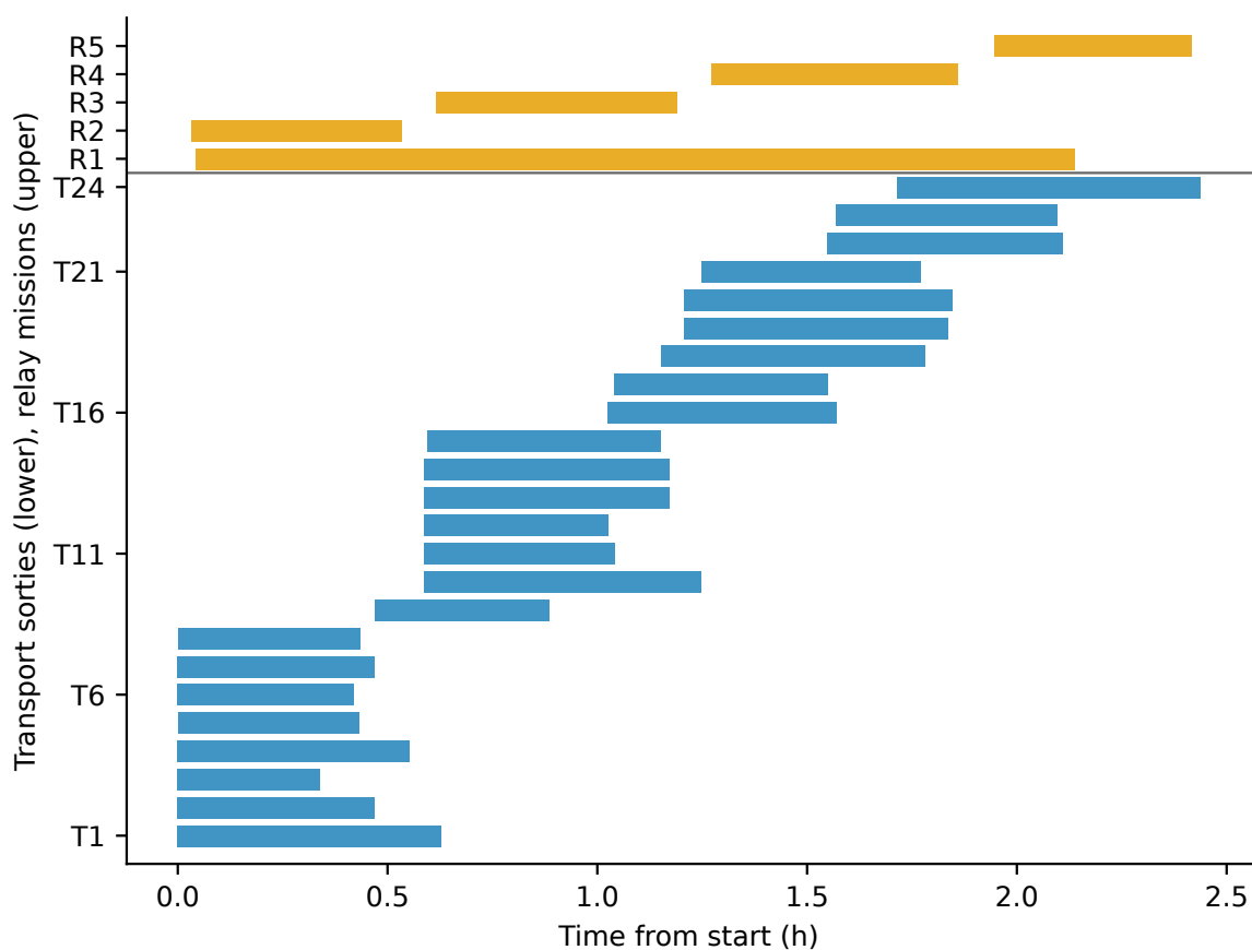
图 5.8 第三问运输与中继任务的联合时间安排; T1-T24 为运输架次, R1-R5 为中继架次
