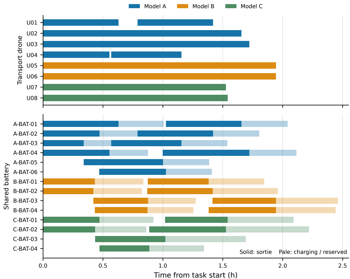
图 4.2 问题二正式方案的运输机与共享电池占用时间轴；浅色部分为返航后的电池充电和保守预留区间
