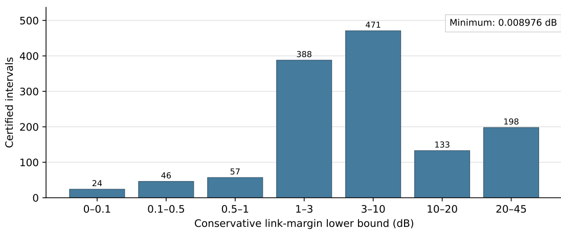
图 4.10 问题三连续通信证书的保守链路裕量下界分布；各柱为已证区间数量，非独立实验重复次数
