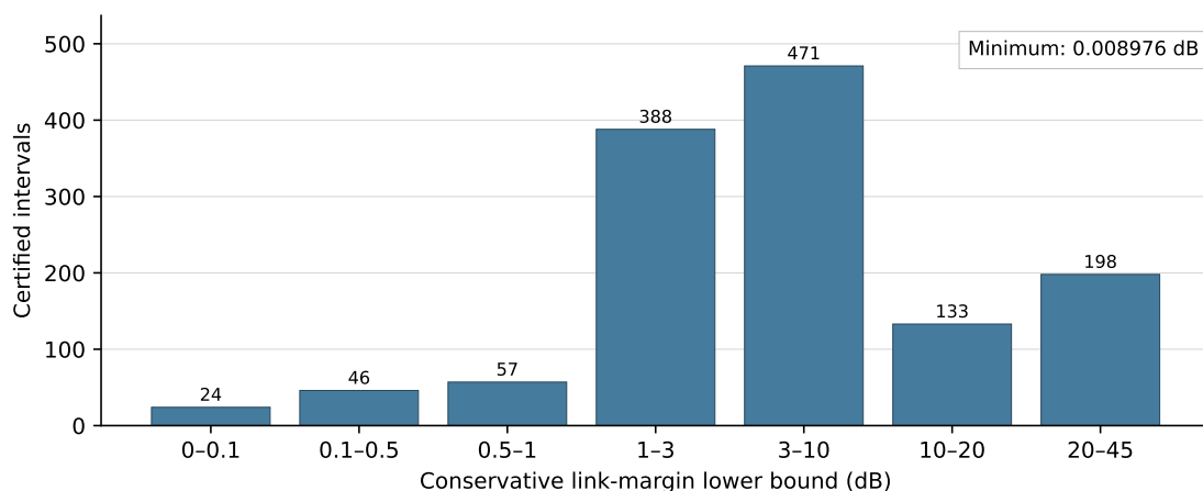
图 7.12 问题三连续通信证书的保守链路裕量下界分布；各柱为已证区间数量，非独立实验重复次数
