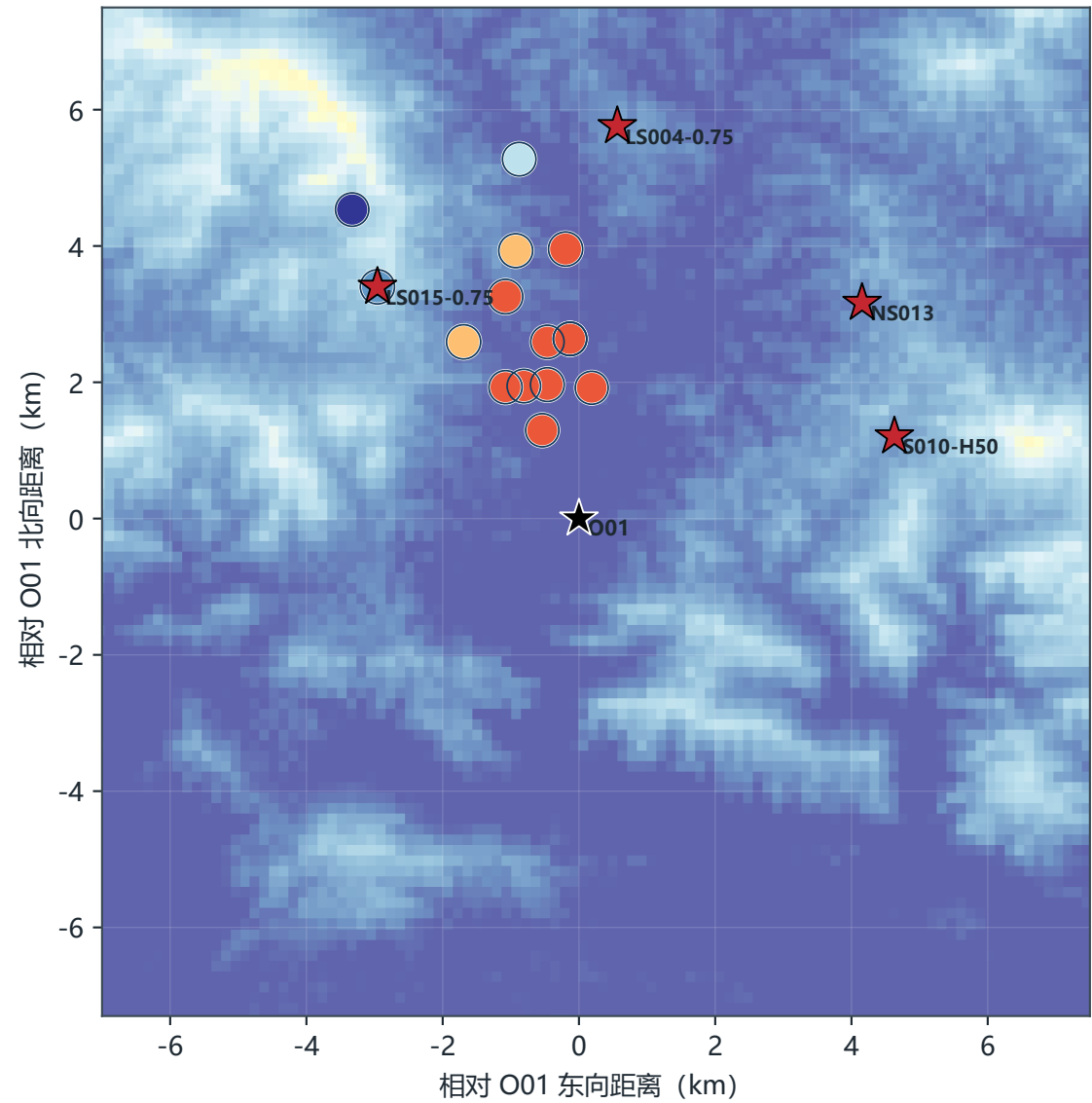
a 候选中继点与最终任务位置
