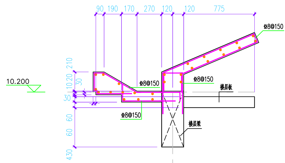
1 檐口大样图 未注明的分布点筋均为 \Phi 8
