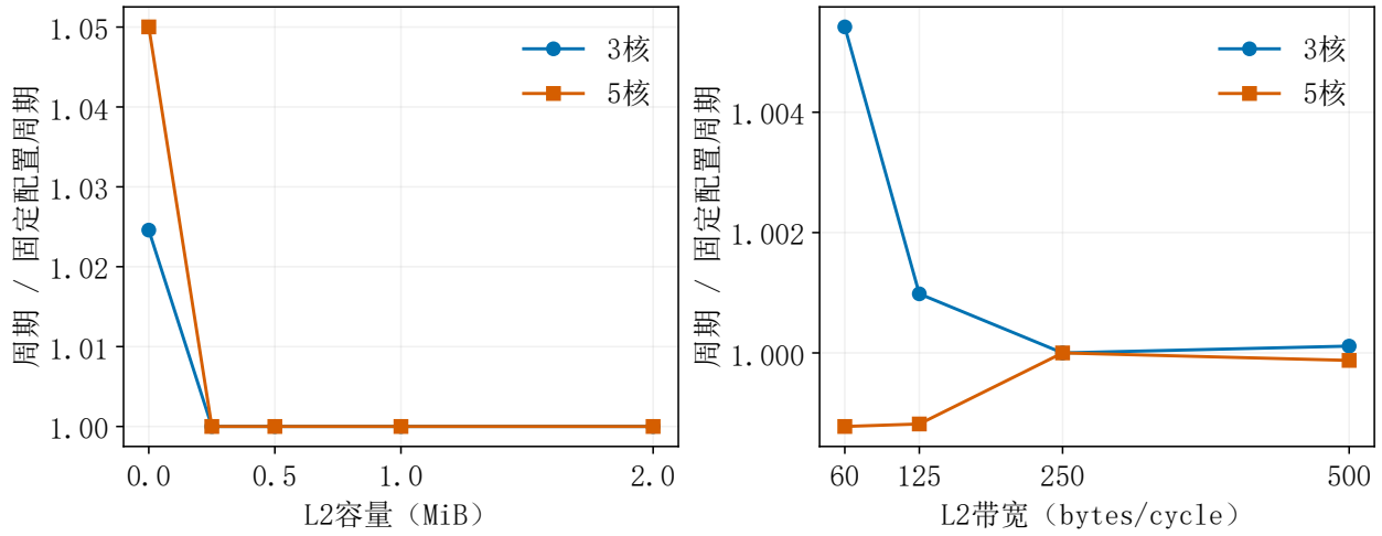
图 4: case005 固定方案的容量与带宽诊断，分母为固定配置周期
