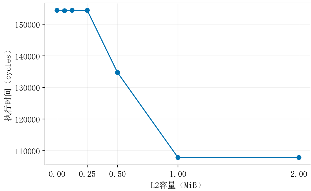
图 3: case044 单核的容量影响: 收益来自 spill reload 命中
