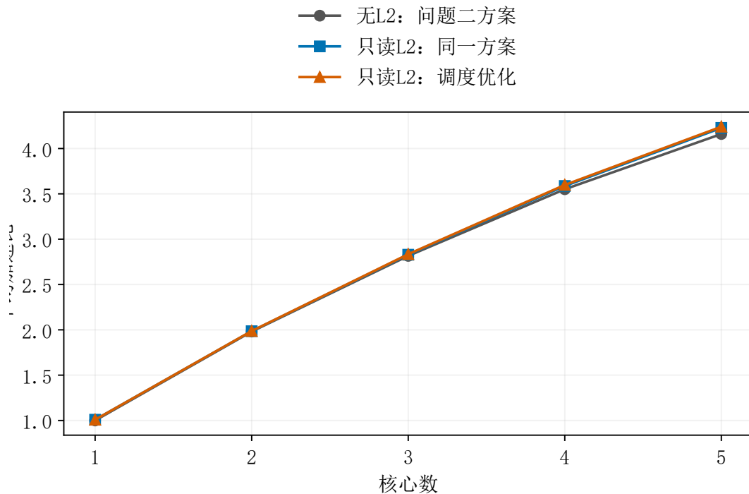
图 1: 无 L2 与只读 L2 的五点加速比对照
