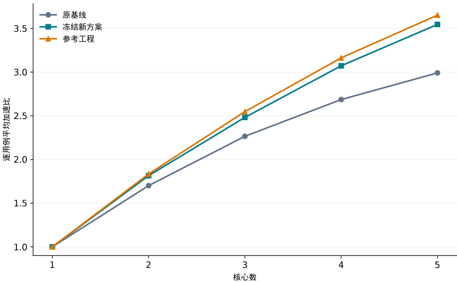
问题一：100个用例的平均加速比
