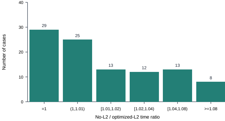
图 7 问题三五核同图同核无 L2 与优化 L2 的时间比直方图
