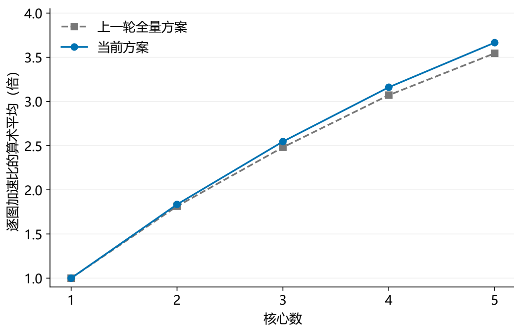
图 1 问题一的百图逐图加速比算术平均
