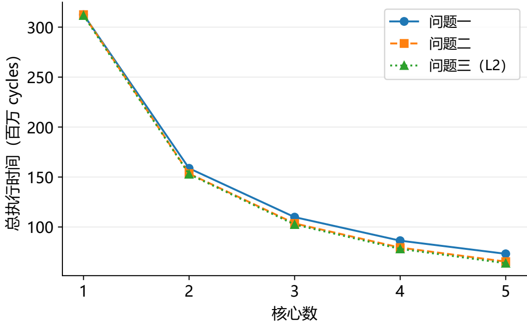
图 4 三问百图总周期；与逐图平均加速比采用不同权重
