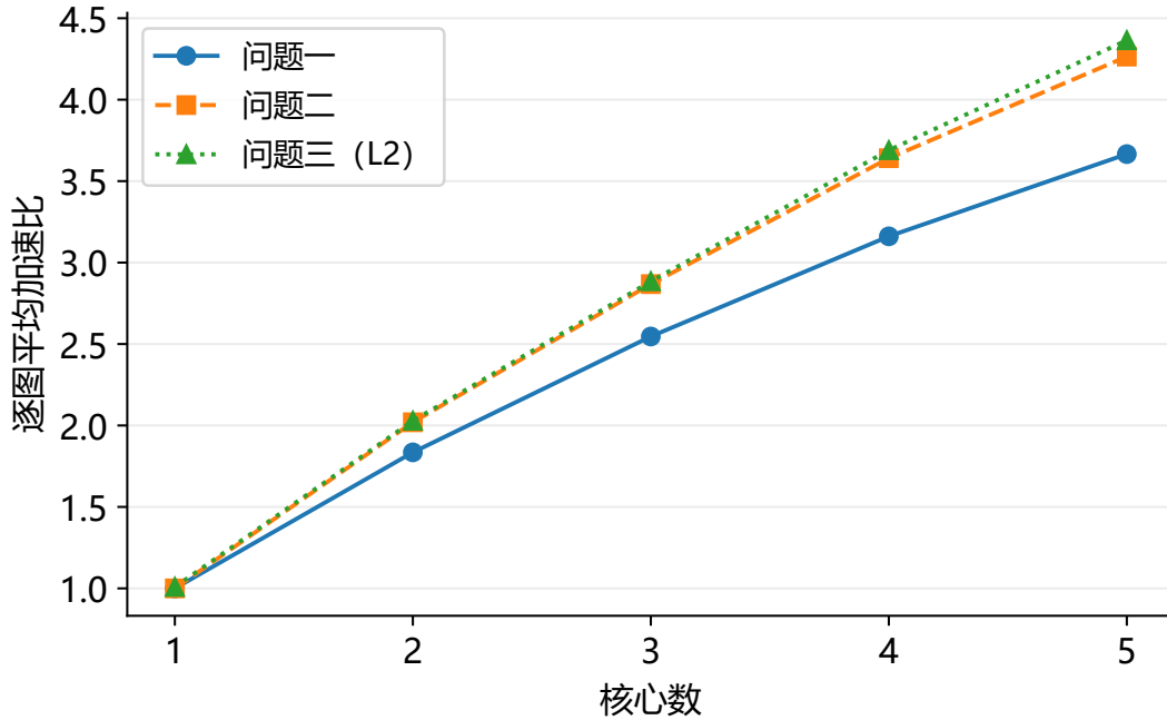
图 3 三问的百图逐图平均加速比；L2 单核点沿用无 L2 单核参考
