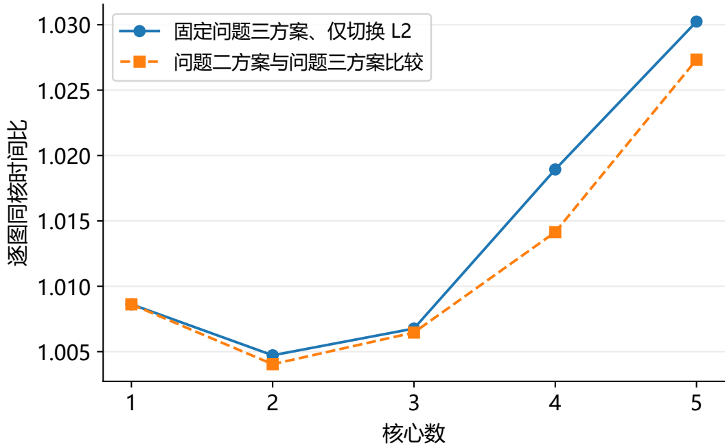
图 5 固定问题三方案的 L2 效应与跨方案综合比较
