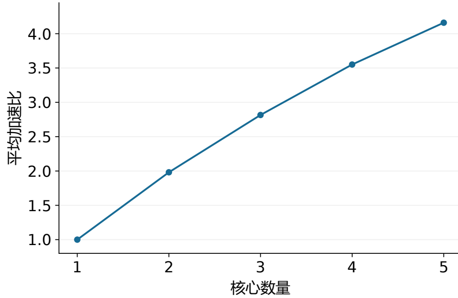
图 1: 场景 B 下 100 个算例的平均加速比，按规定单核基准与各核执行周期之比逐例取算术平均。
