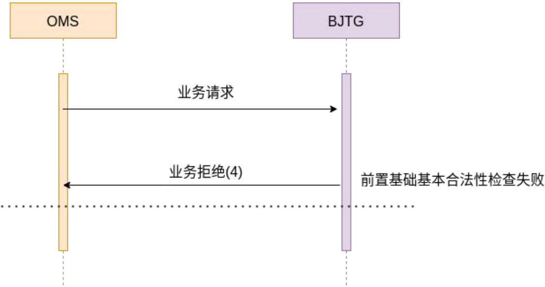
图 3-1 业务拒绝消息流示意图
