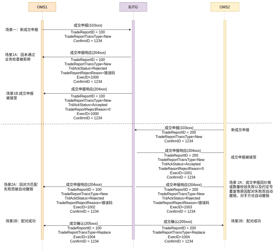
图 3-11 新成交申报处理消息示意图
