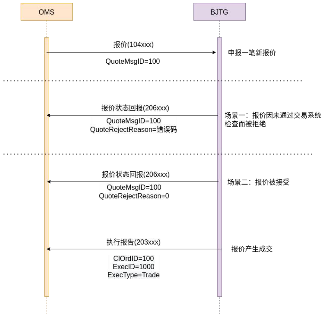
图 3-4 新报价处理消息流示意图
