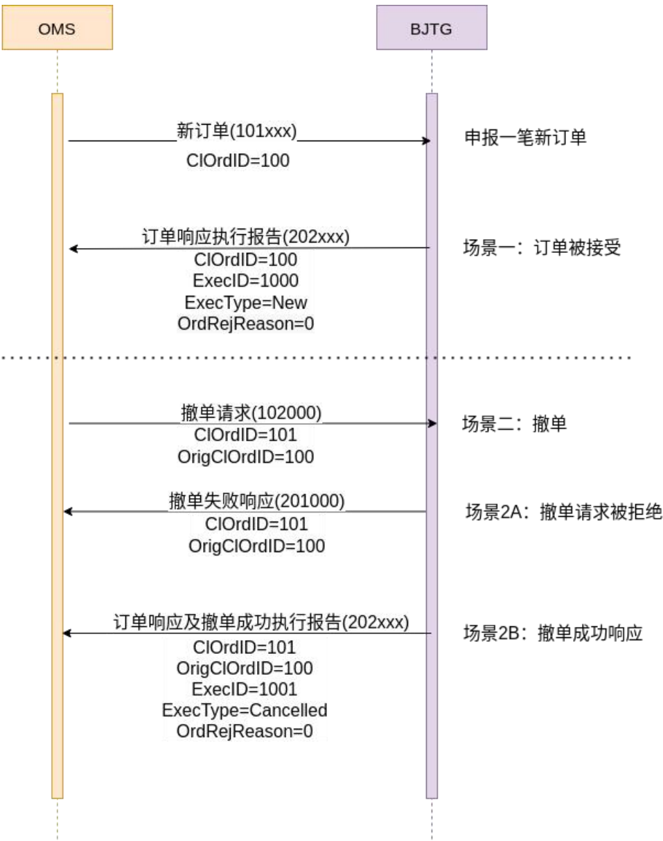
图 3-3 撤单请求消息流示意图
