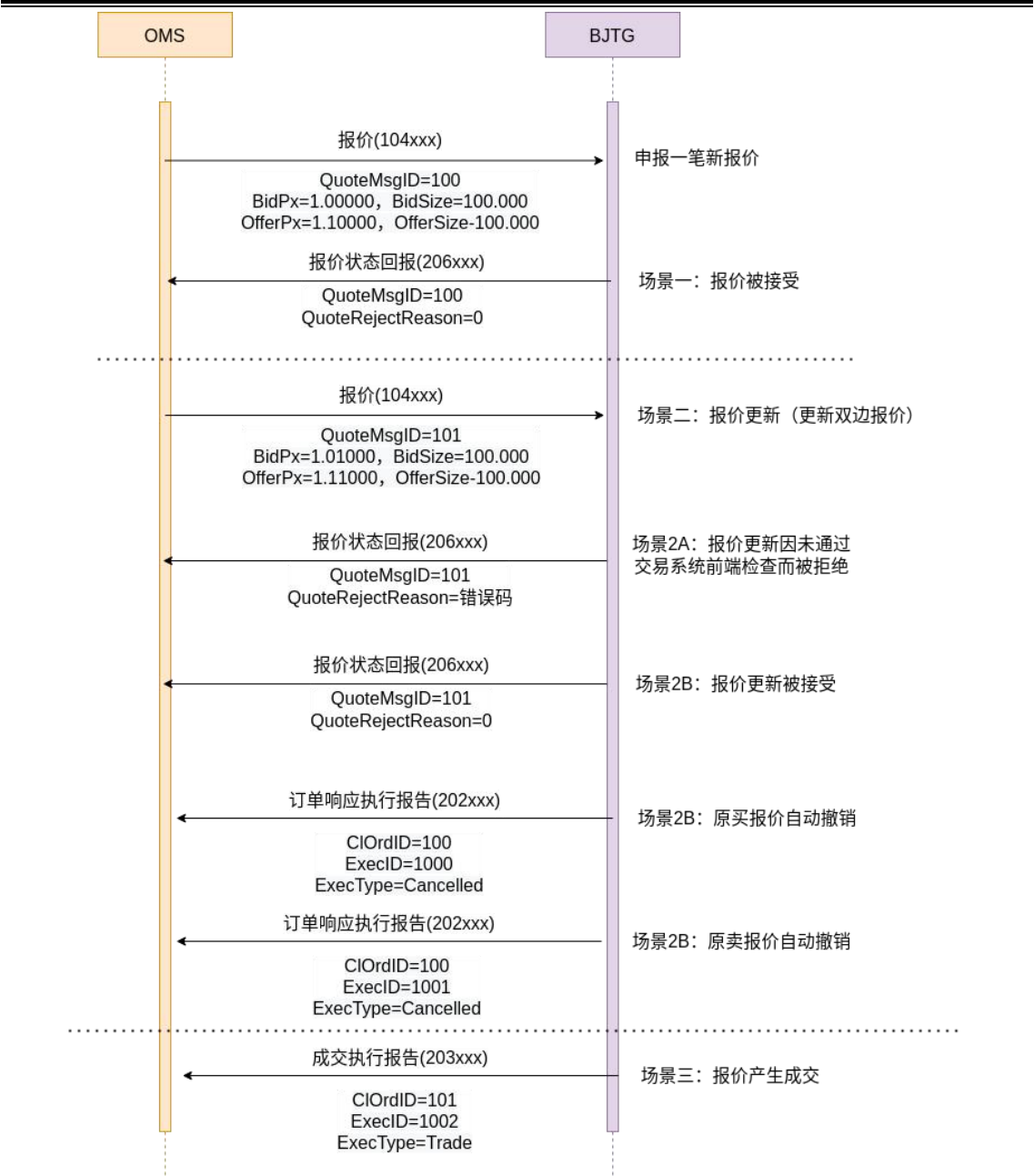
图 3-5 更新双边报价处理消息流示意图
