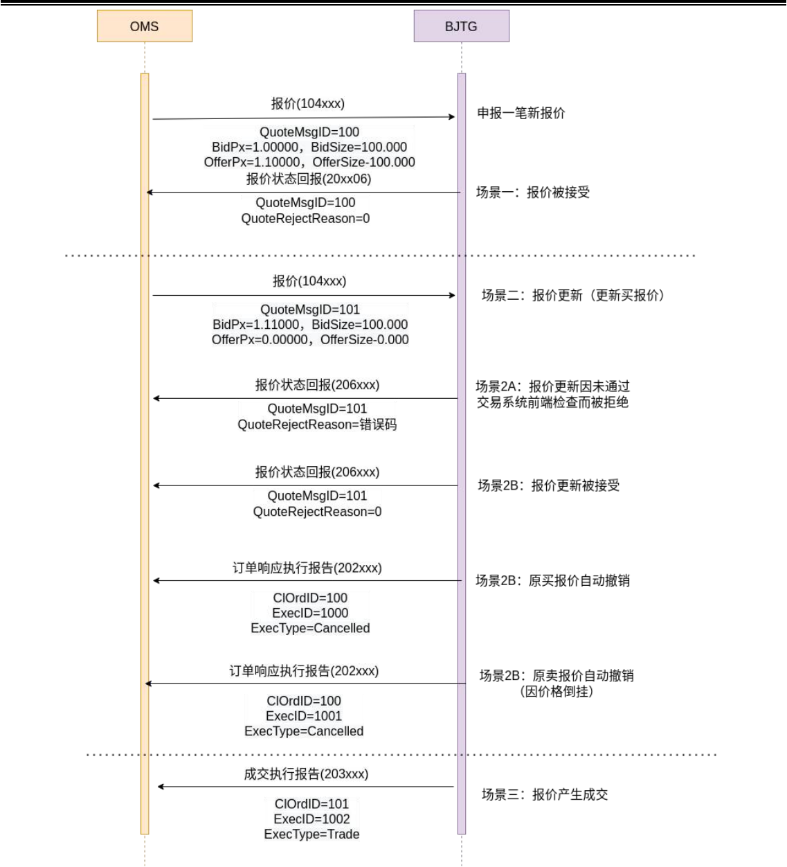
图 3-7 更新单边报价（情形三）处理消息流示意图
