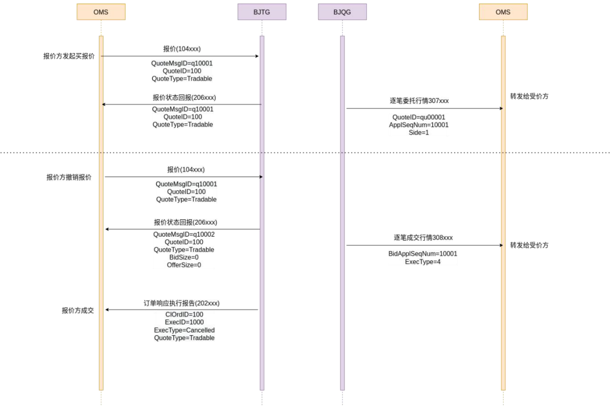
图 3-10 报价方撤销报价处理消息流示意图
