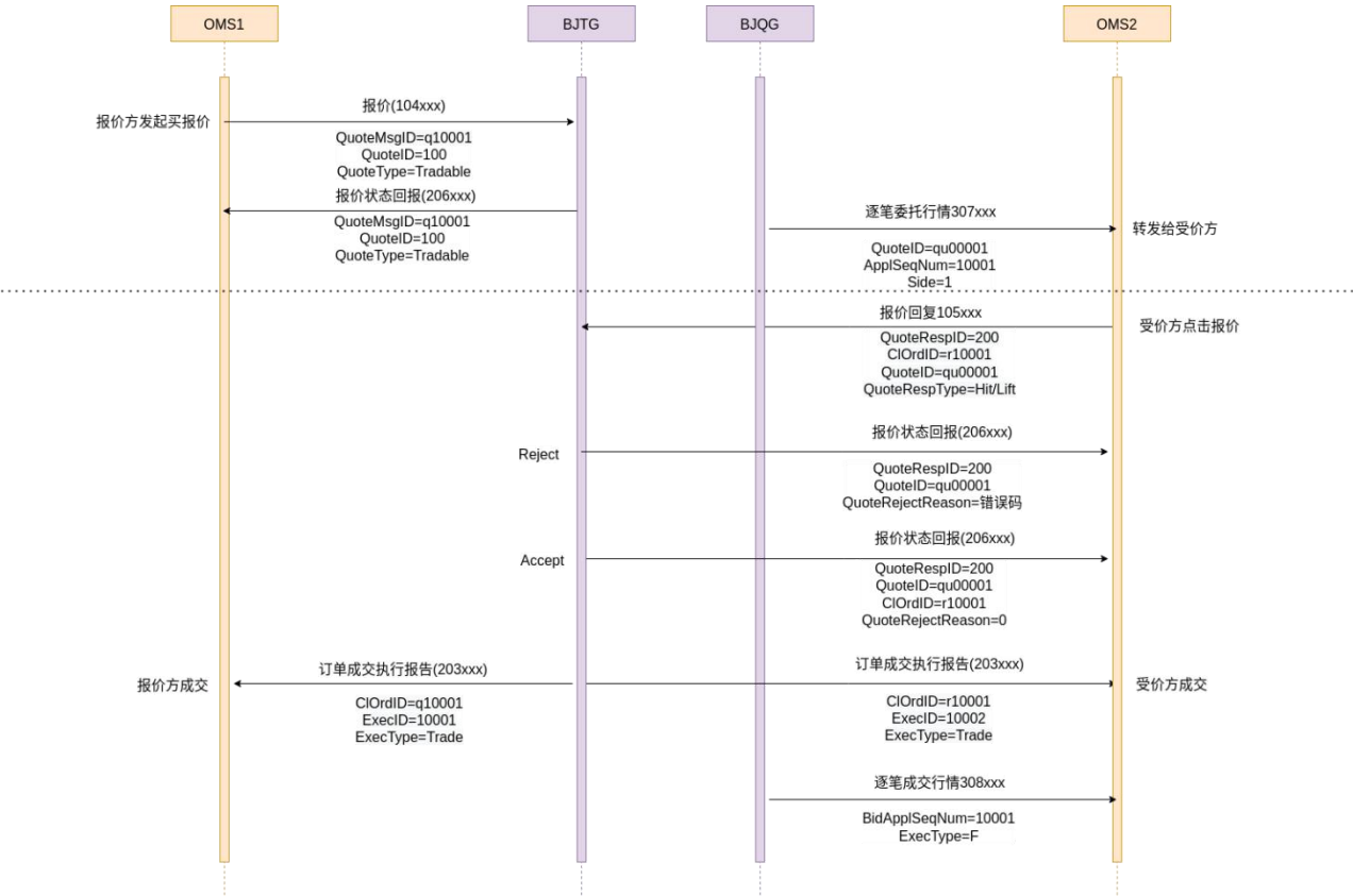
图 3-9 受价方点击成交处理消息流示意图
