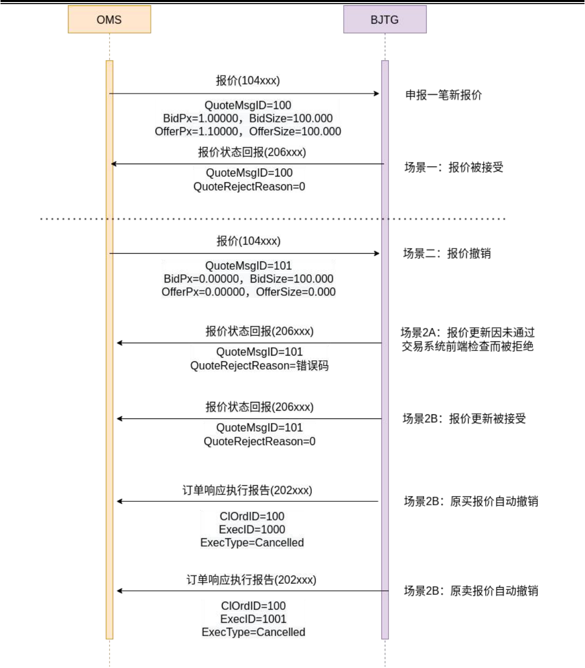
图 3-8 报价撤销处理消息流示意图
