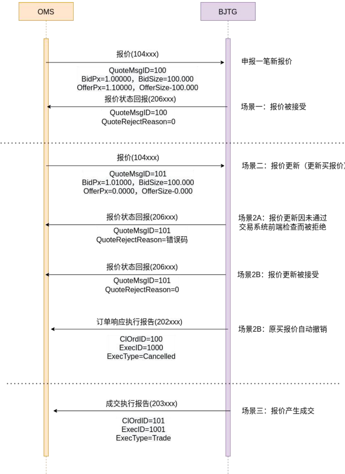
图 3-6 更新单边报价（情形二）处理消息流示意图
