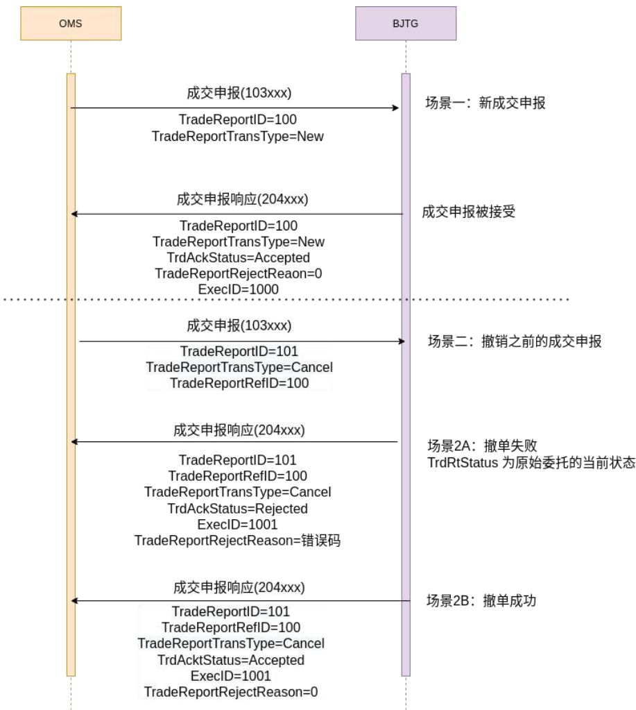
图 3-12 撤销成交申报处理消息流示意图
