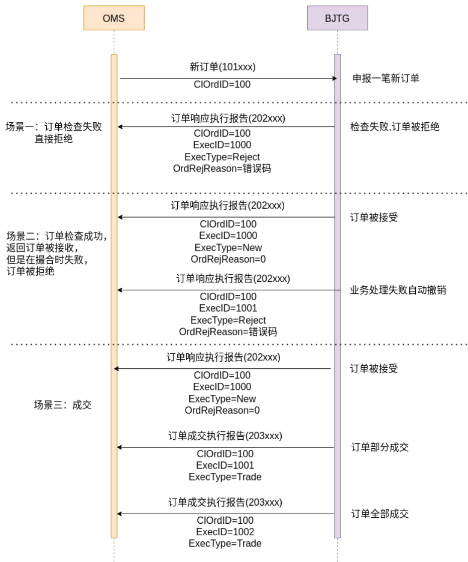
图 3-2 新订单消息流示意图
