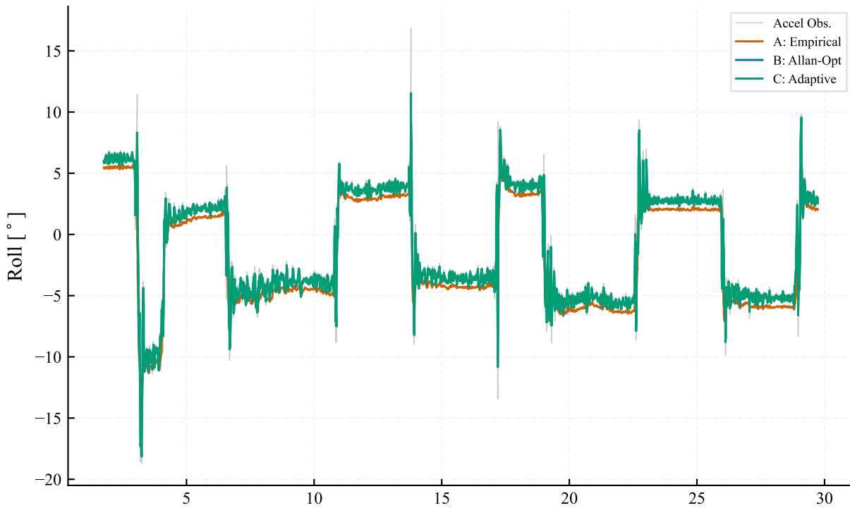
Roll: KF Estimate
