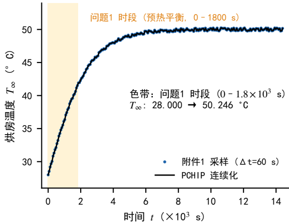
(a) 烘房温度 (附件1)
