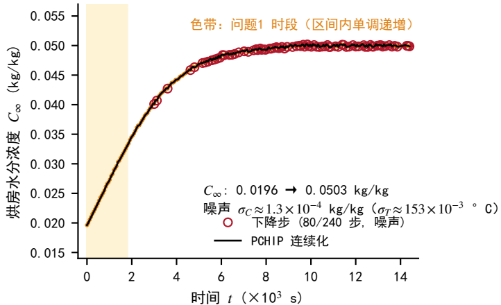
(b) 烘房水分浓度 (附件1, 含测量噪声)
