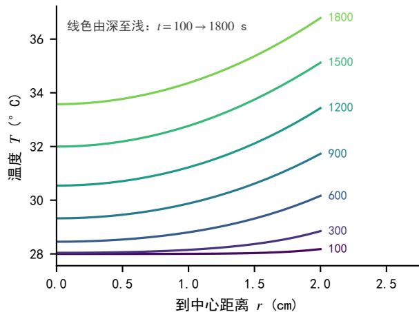
(c) 温度径向剖面 (表1 时刻)
