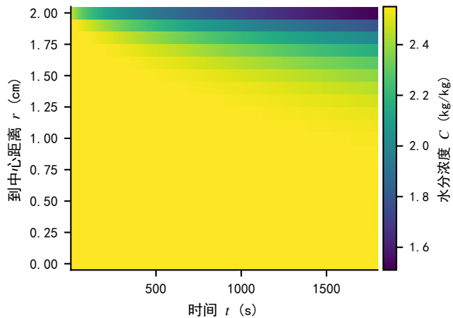
(d) 水分浓度径向剖面 (表2 时刻)
