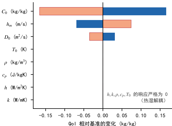
(c) 表面水分 C(R, t_{end})
