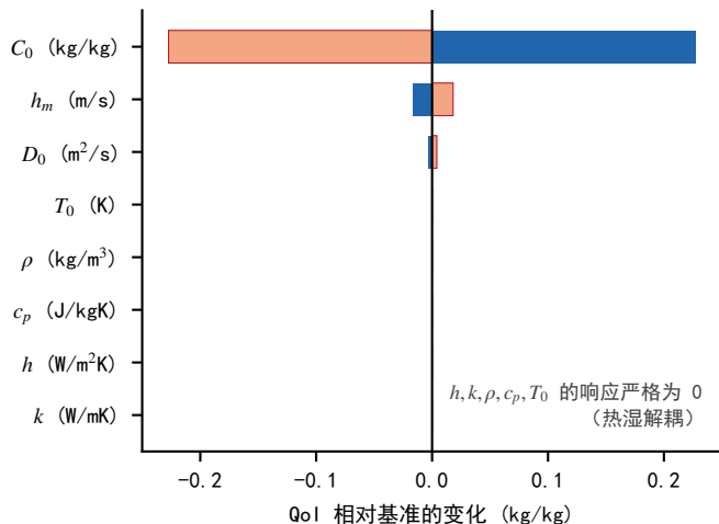
(d) 体积平均水分 \langle C \rangle(t_{end})
