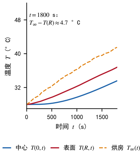
(c) 中心/表面温度演化与烘房环境
