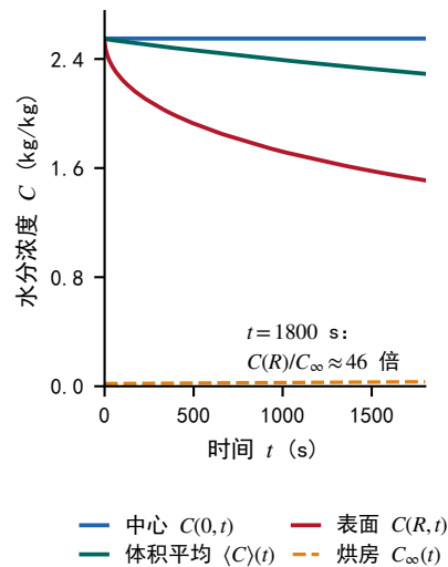
(f) 各层浓度演化与体积平均
