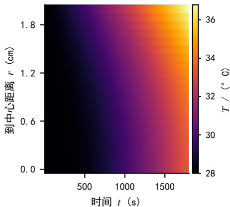
(a) 温度场时空热图 T(r, t)
