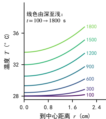
(b) 径向剖面 (表1 时刻)
