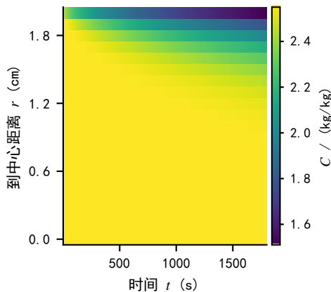
(d) 水分浓度场时空热图 C(r, t)
