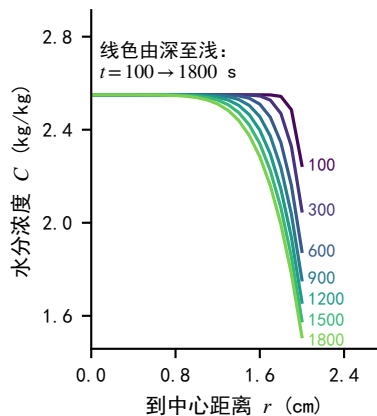
(e) 径向剖面 (表2 时刻)
