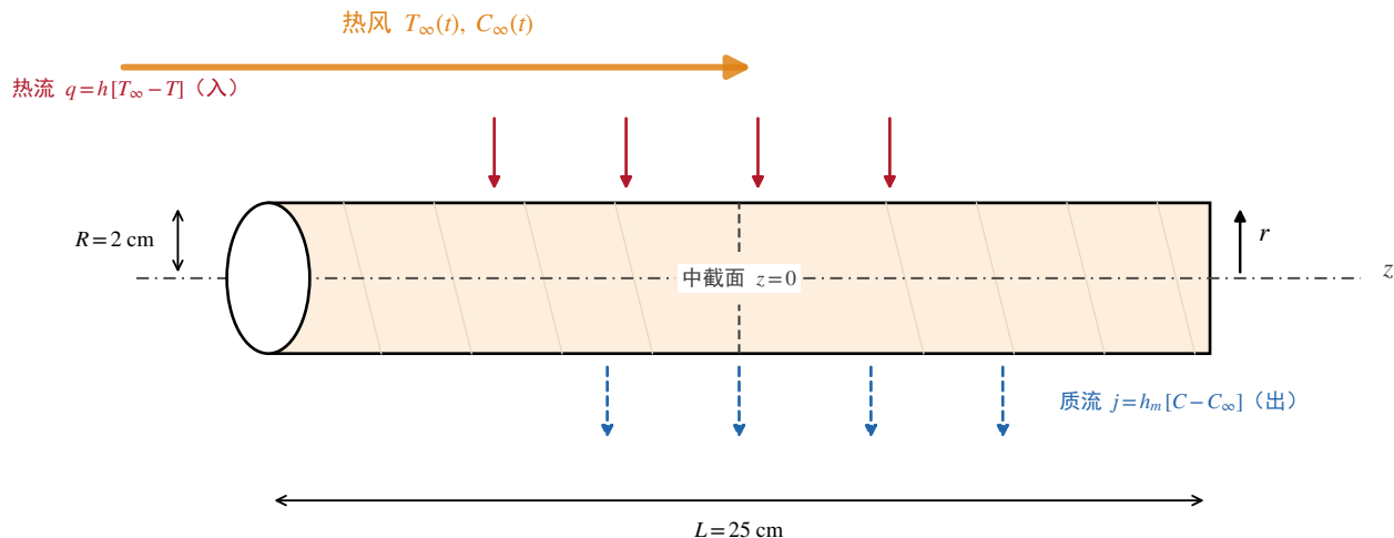
(a) 物理模型：圆柱药材与第三类边界条件
