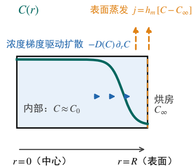
(c) 水分径向扩散示意
