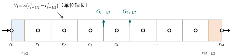
(b) 一维径向求解域与节点式有限体积 (图示 M=8 )
