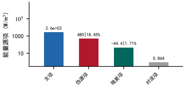
(b) 能量源项量级
