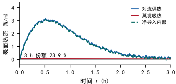
(c) 表面热流分解
