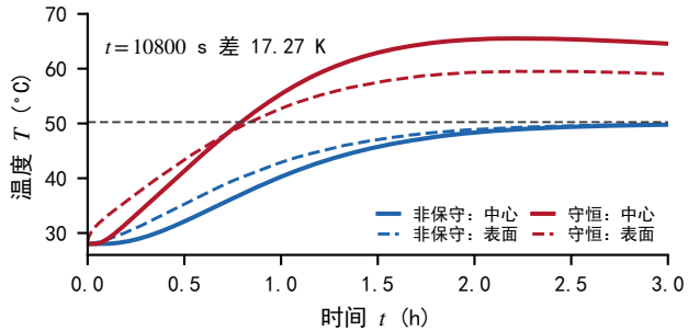
(a) 两种写法的温度演化
