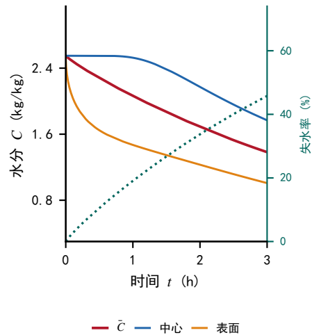
(f) 分层演化与失水率
