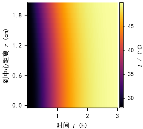
(a) 温度场 T(r, t)
