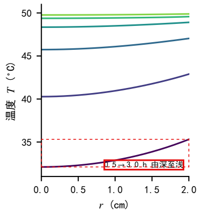
(b) 温度径向剖面
