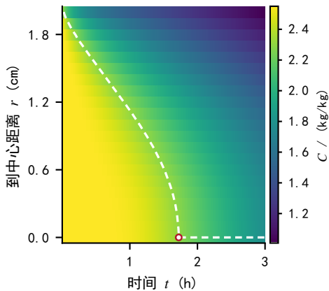
(d) 水分场与干燥前沿
