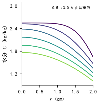
(e) 水分径向剖面
