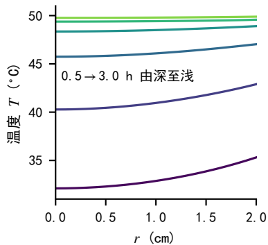
(b) 温度径向剖面
