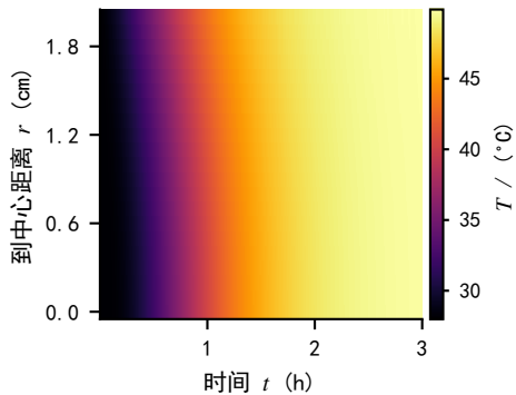
(a) 温度场 T(r, t)
