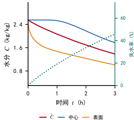
(f) 分层演化与失水率
