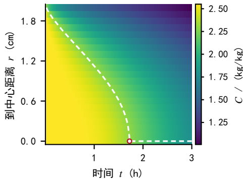
(d) 水分场与干燥前沿
