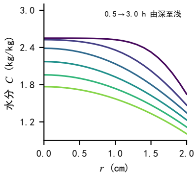
(e) 水分径向剖面
