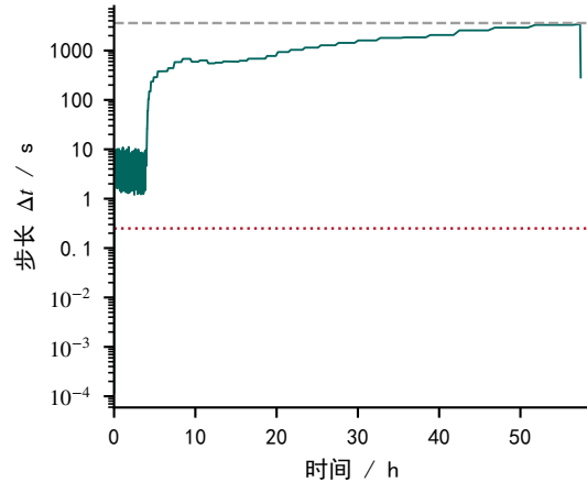
(c) BDF 步长演化
