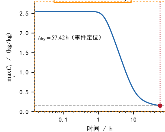
(a) 全场最大含水率 \max_i C_i(t)
