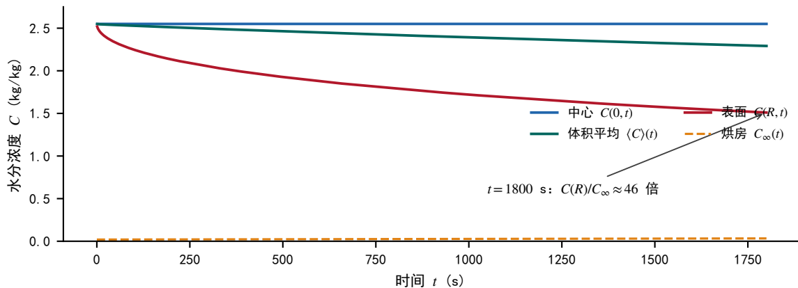
(c) 各层浓度演化与环境对比: 仅表层脱湿, 表面远未平衡
