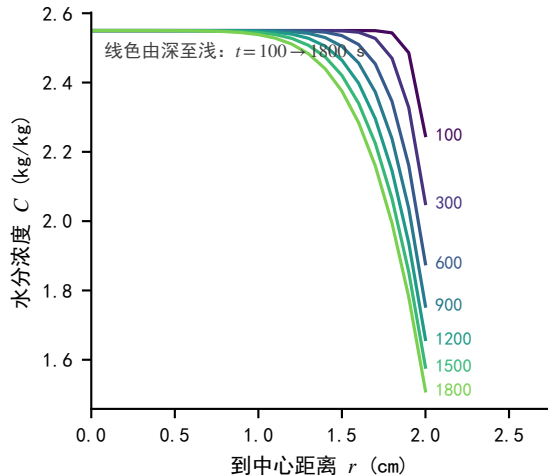
(b) 径向剖面 (表2 时刻)
