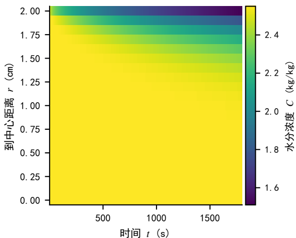
(a) 水分浓度场时空热图 C(r, t)
