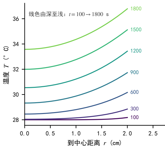
(b) 径向剖面 (表1 时刻)
