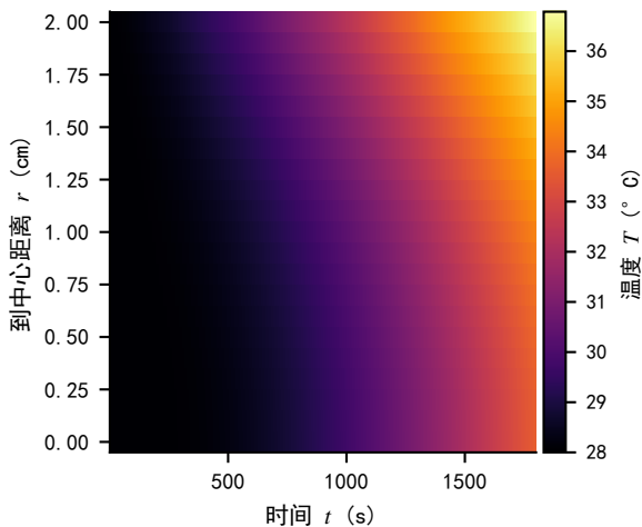
(a) 温度场时空热图 T(r, t)
