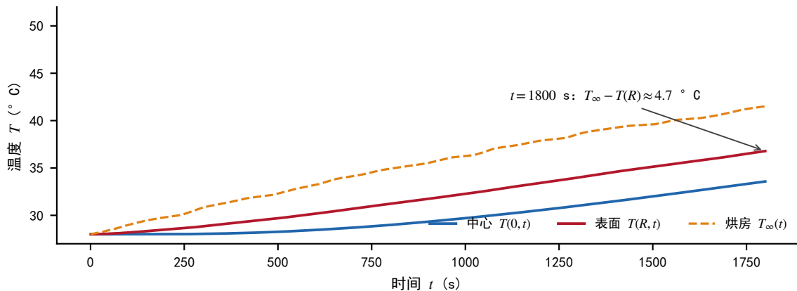
(c) 中心/表面温度演化与烘房环境对比：三级滞后，预热未完成
