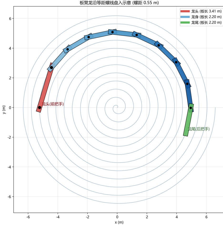
图 1 板凳龙沿等距螺线盘入的几何结构局部示意图
