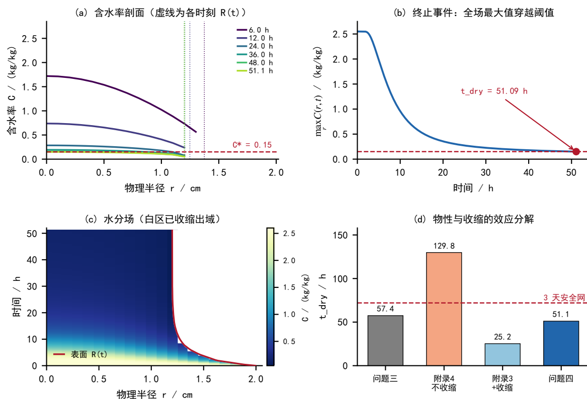
图 12 问题四的主要结果。(a) 含水率剖面随收缩推进，点线标出各时刻的表面位置，水分自表面向内依次降低；(b) 终止事件，全场最大含水率单调下降到阈值，事件函数在末 2h 无回升，说明单根；(c) 物理坐标下的水分场，白色区域是已收缩出域的部分，可见表面积在 36 h 后基本冻结在 1.20 cm；(d) 物性与收缩的效应分解。
