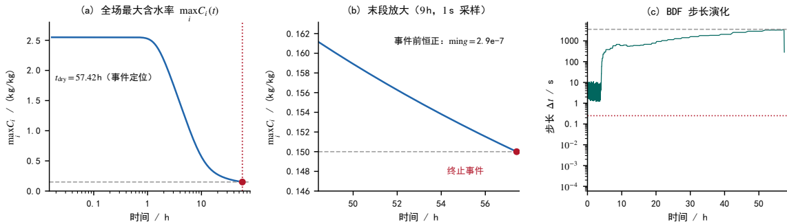
图 8 烘干时间的确定。(a) 全场最大含水率的演化：与阈值（虚线）的唯一交点即 t_{\text{dry}} （红点）；(b) 末段 9h 放大（1s 采样）：事件前 g = \max_i C_i - C^* 恒正、终点为零；(c) BDF 步长演化：虚线为步长上界 3600 s，点线为问题二定步长 0.25 s。
