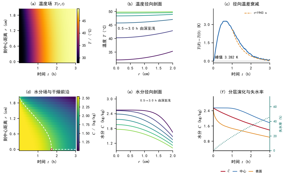
图 7 问题二温度场与水分浓度场结果。(a) 温度场时空热图；(b) 温度径向剖面；(c) 径向温差先增后减并趋于准均匀；(d) 水分浓度场时空热图与干燥前沿轨迹（白色虚线为 C = 2.295 \text{ kg/kg} 等值线，圆点为前沿抵达中心时刻 t = 6204 \text{ s} ）；(e) 水分径向剖面；(f) 中心、表面与体积平均含水率及累计失水率（点线，右轴）。
