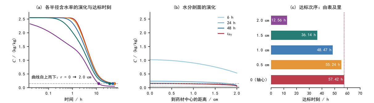
图 9 由表及里的达标次序。(a) 五个输出半径的含水率演化，圆点为各自达到 C^* 的时刻；(b) 水分剖面的演化（6、24、48 h 与 t_{\text{dry}} ），虚线为阈值 C^* = 0.15 ，点线为环境平台值 0.0500；(c) 达标时刻随半径的分布：由表及里，轴心最后达标。
