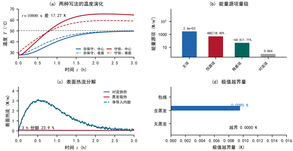
图 6 能量方程形式与蒸发吸热的作用。(a) 两种写法的中心/表面温度演化：守恒形式在 t = 10800 s 给出中心温度 64.5646^\circ\text{C} ，超出烘房温度峰值 50.2460^\circ\text{C} （点划线）；(b) 四个能量源项的量级，守恒形式伪源项占主项 18.45%、严格方程的自洽极限下残余项为零；(c) 表面热流分解；(d) 极值原理越界量。
