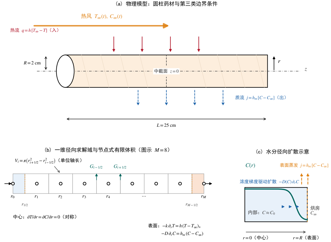
图 3 问题一的物理模型与离散。 a 圆柱药材的第三类边界（热风对流换热与对流传质）与中截面； b 一维径向求解域的节点式有限体积网格与控制体（图示 M = 8 ）； c 水分在浓度梯度驱动下向表面输运并蒸发。
