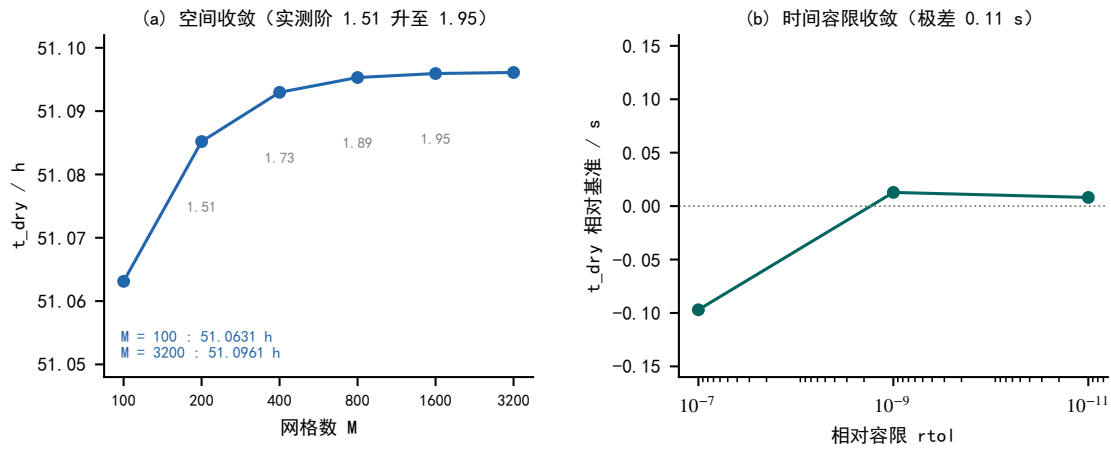
图 13 数值收敛性。(a) 网格由 100 加密到 3200，实测收敛阶由 1.51 逐级升到 1.95，即该格式的渐近阶为二阶；(b) 相对容限由 10^{-7} 收紧到 10^{-11} ，烘干时间的极差仅 0.11 s，时间积分已完全收敛。
