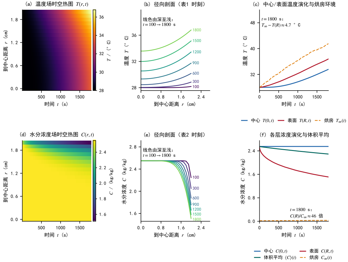
图 4 问题一的结果。上排温度场： a 时空热图； b 表 1 时刻的径向剖面； c 中心/表面温度演化与烘房环境对比。下排水分浓度场： d 时空热图； e 表 2 时刻的径向剖面； f 各层浓度演化与体积平均。
