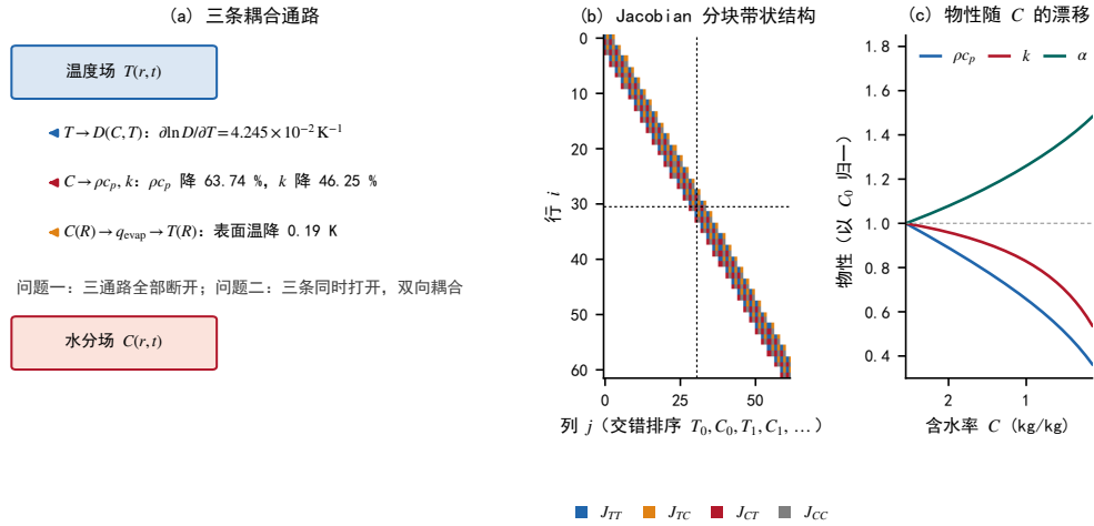
图 5 问题二的耦合结构。(a) 三条耦合通路（对照问题一三通路全部断开）；(b) Jacobian 分块带状结构（ M = 30 ，非零元 364 个、占 9.47%，四个分块各 91 个）；(c) \rho c_p 、 k 、 \alpha 随含水率 C 的漂移（以 C_0 = 2.55 归一）。
