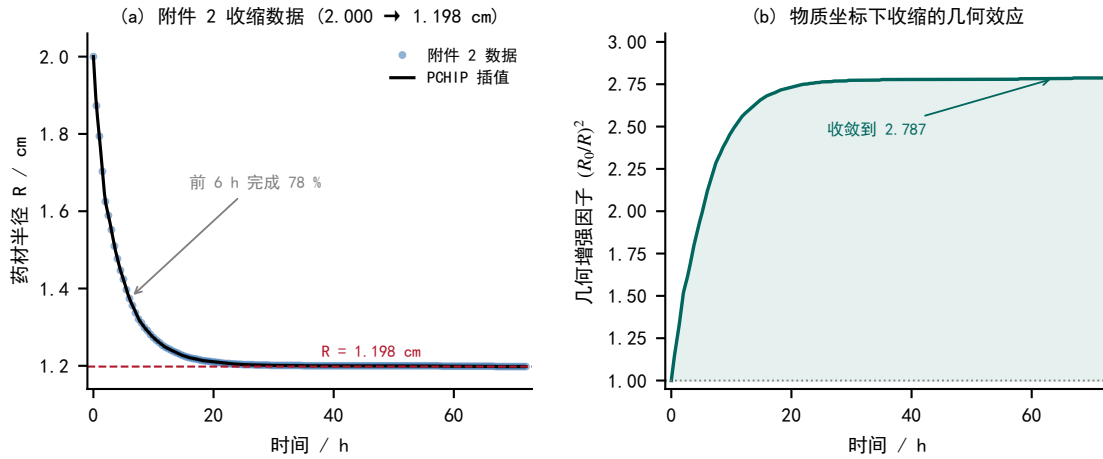
图 11 收缩数据与几何效应。(a) 附件 2 的半径序列呈两段式：前 6 h 完成全部收缩量的 78%，此后趋于饱和，全程严格单调；(b) 物质坐标下收缩的全部效应归结为几何因子 (R_0/R)^2 ，它由 1 升到 2.79，即内部再分布被加快近三倍。
