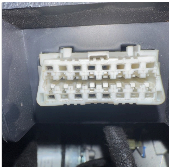
OBD插接件
