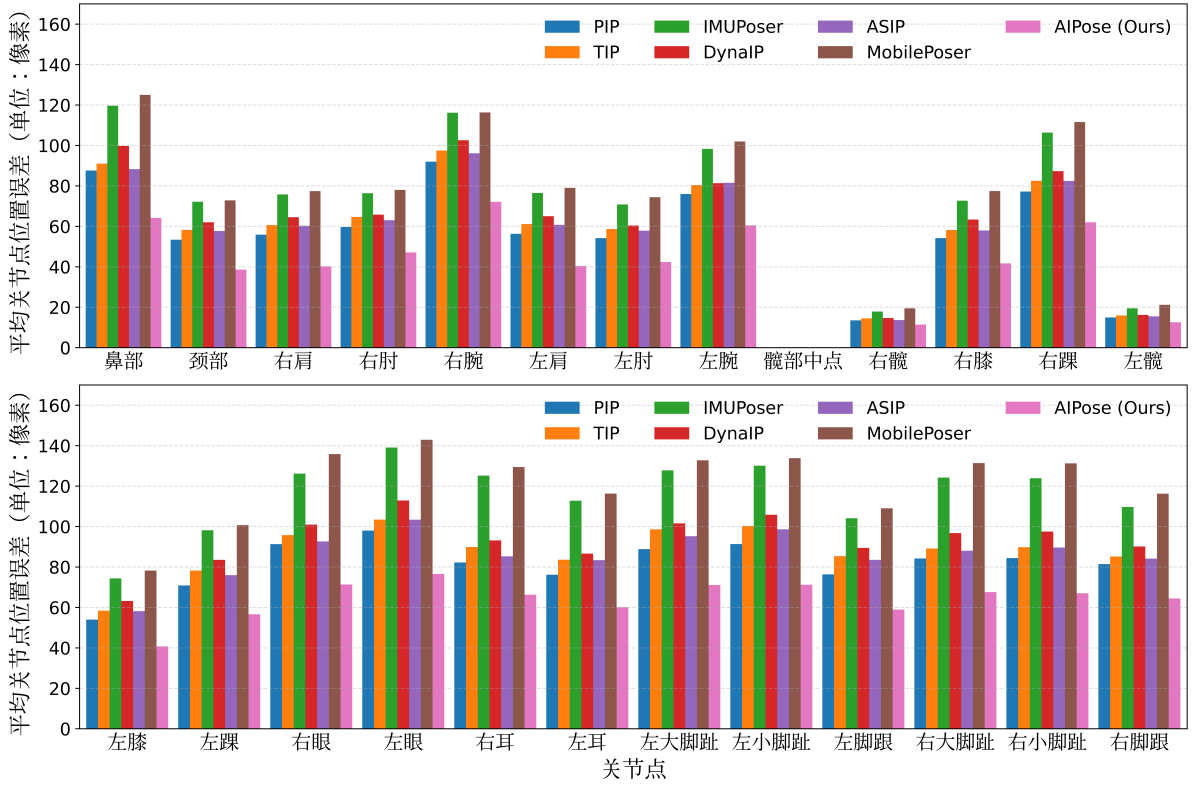
图 4-7 不同方法在当前姿态重构任务中各关键点的 MPJPE
