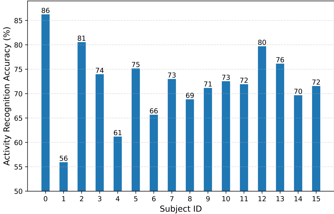
图 3-9 跨受试者活动识别准确率
