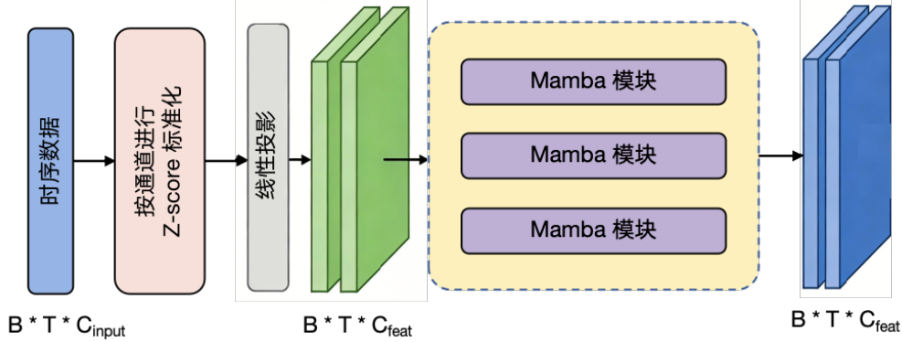
图 3-3 Mamba 特征编码器
