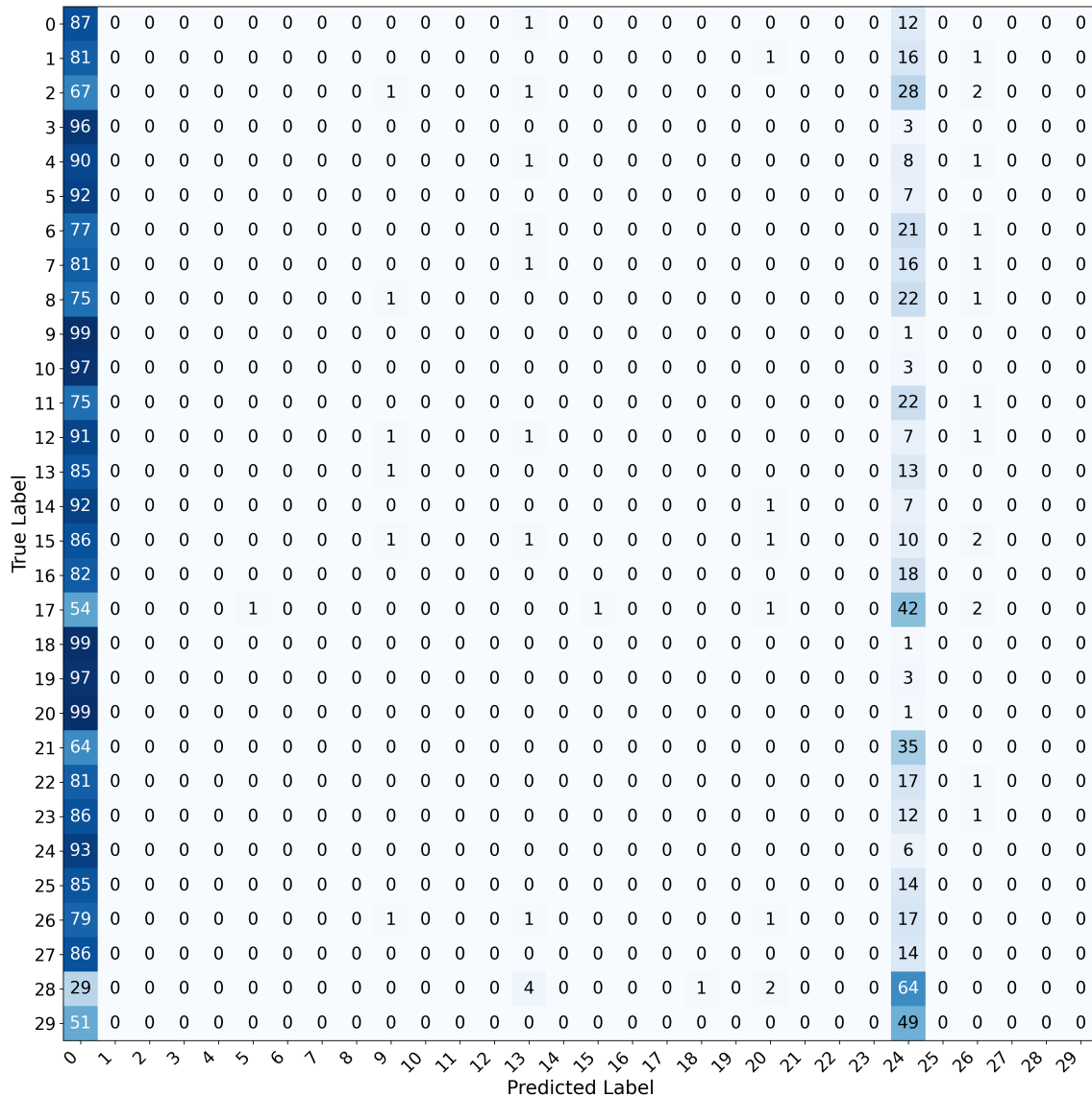
图 3-10 采用按通道 Z-score 标准化后的活动识别归一化混淆矩阵
