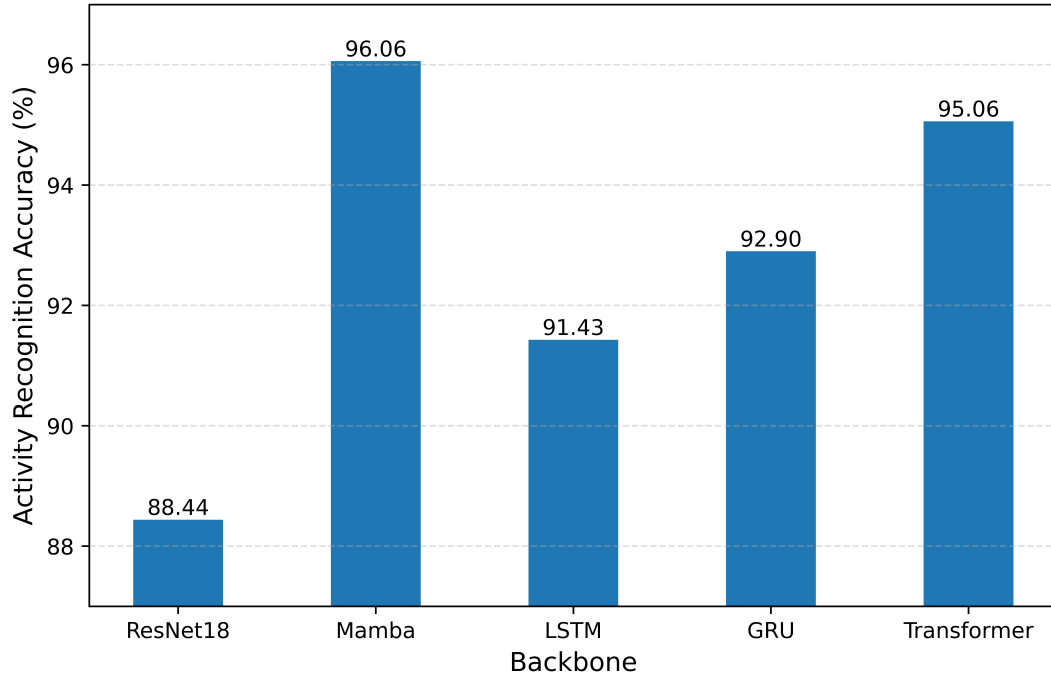
图 3-8 骨干网络选择实验结果
