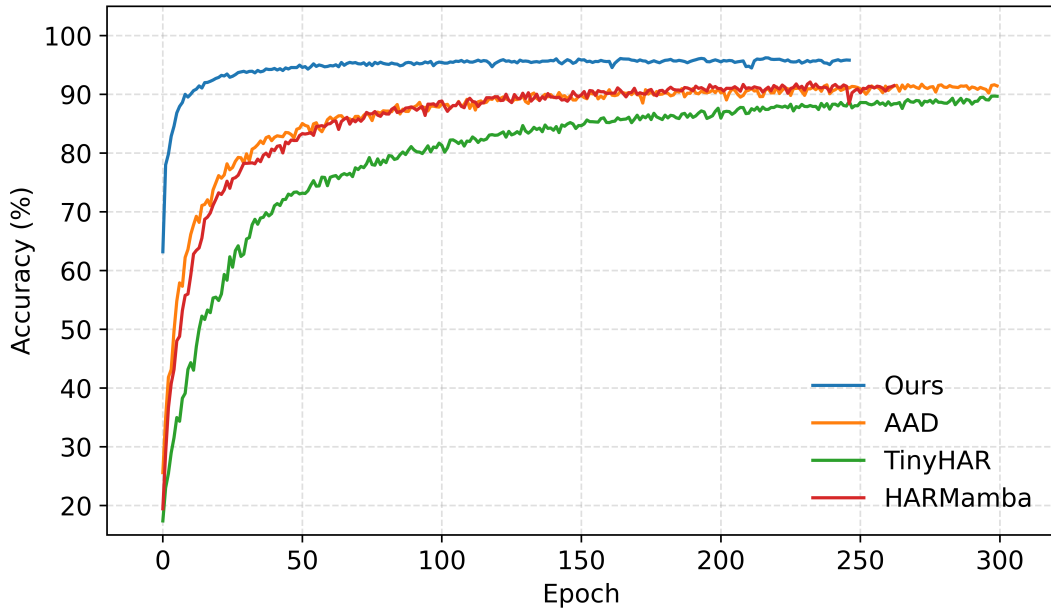
图 3-6 各方法活动识别准确率对比
