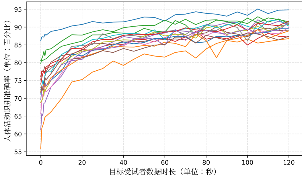
图 3-14 少样本适配条件下的跨受试者活动识别准确率变化
