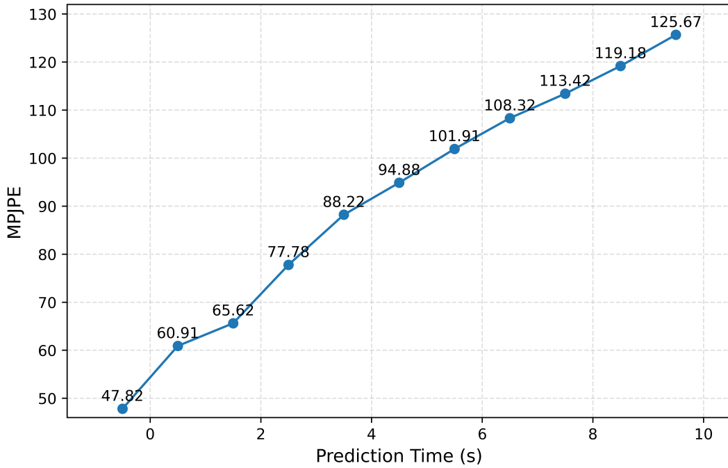
图 4-13 长时姿态预测实验结果
