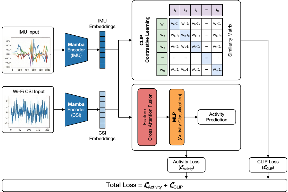
图 3-5 WIHAR 模型架构图
