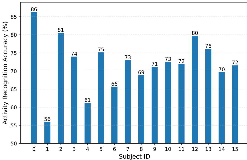
图 3-14 跨受试者活动识别准确率
