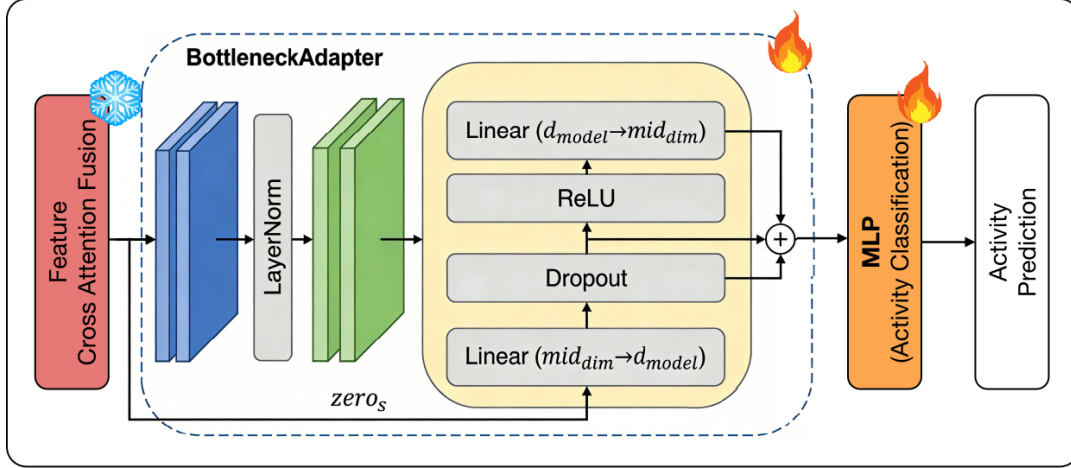
图 3-6 基于瓶颈残差结构的 Adapter 模块示意图
