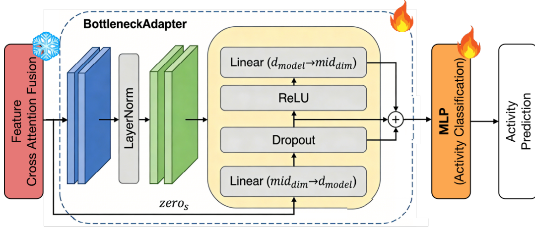
图 3-4 基于瓶颈残差结构的 Adapter 模块示意图
