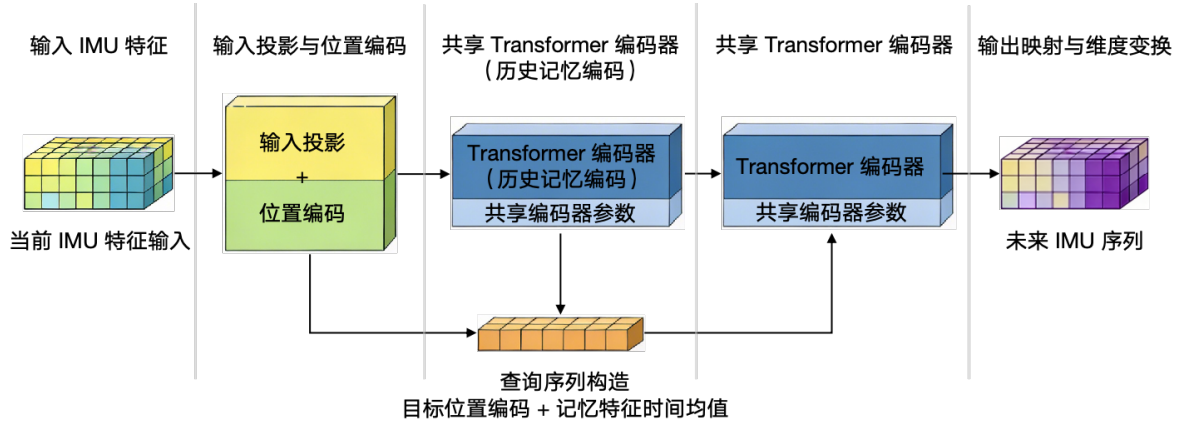
图 4-3 基于共享 Transformer 编码器的 IMU 时序预测模块
