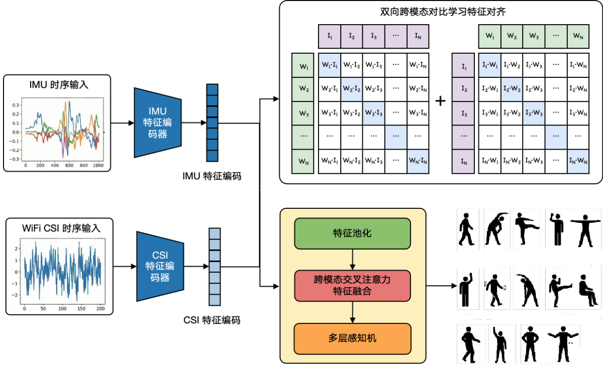
图 3-2 WIHAR 模型架构图
