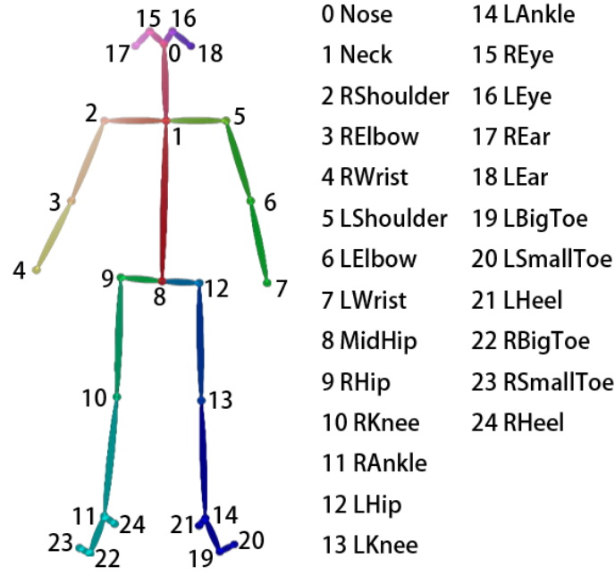
图 4-4 OpenPose 25 点模型
