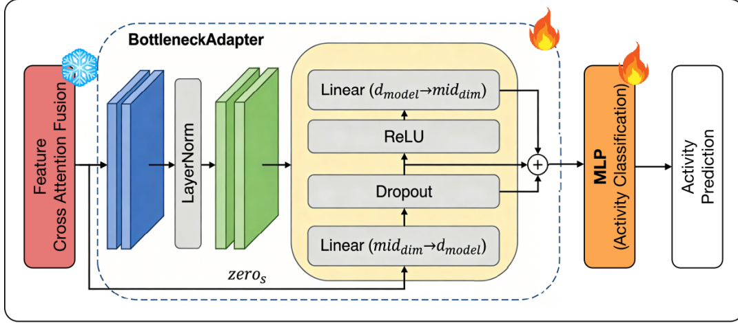
图 3-4 基于瓶颈残差结构的 Adapter 模块示意图
