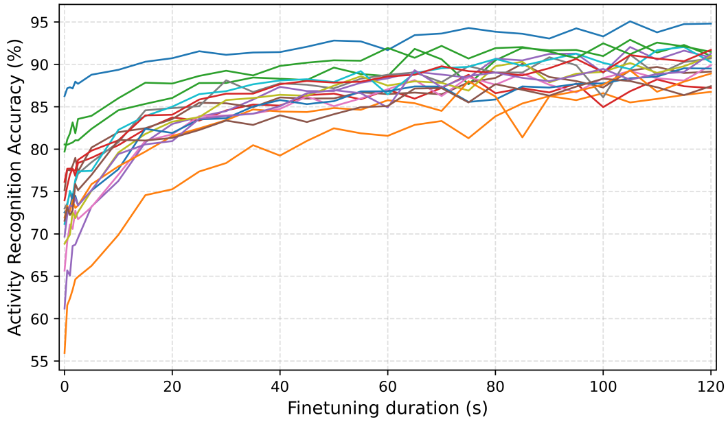
图 3-12 少样本适配条件下的跨受试者活动识别准确率变化
