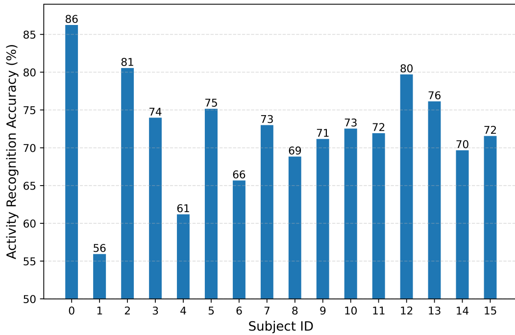
图 3-11 跨受试者活动识别准确率
