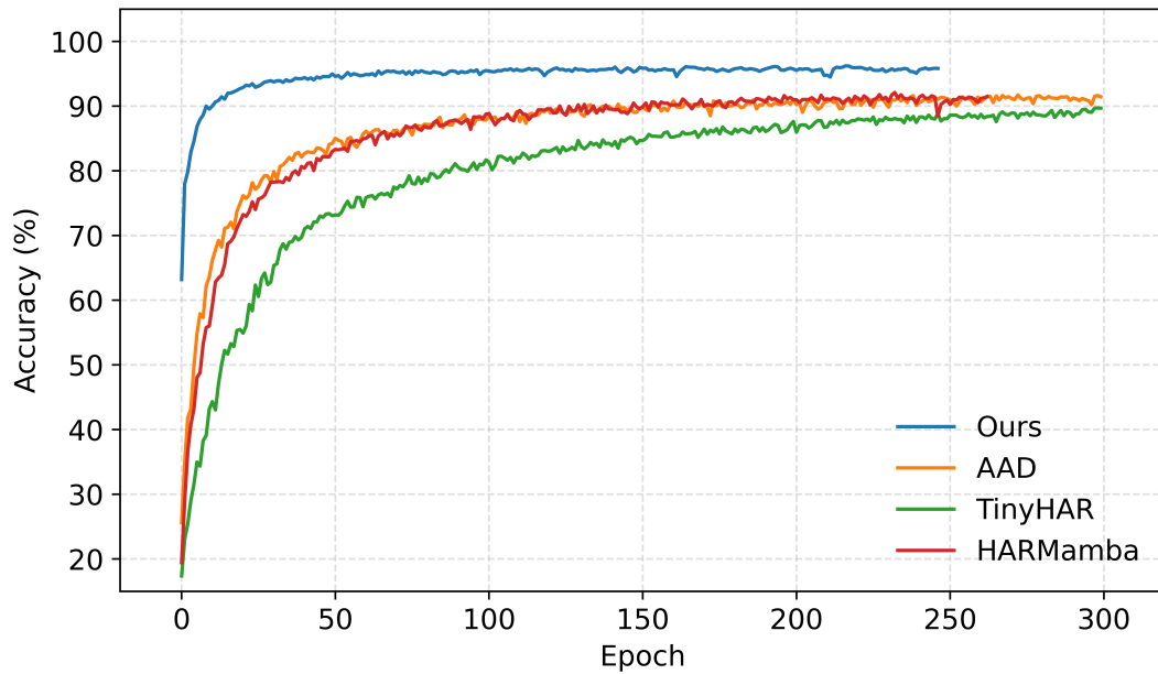
图 3-7 各方法活动识别准确率随训练轮数变化曲线
