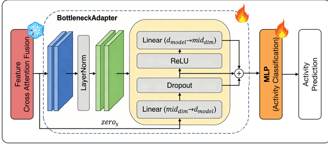
图 3-6 基于瓶颈残差结构的 Adapter 模块示意图
