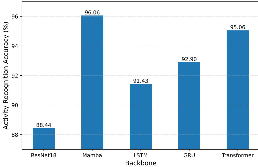
图 3-9 骨干网络选择实验结果
