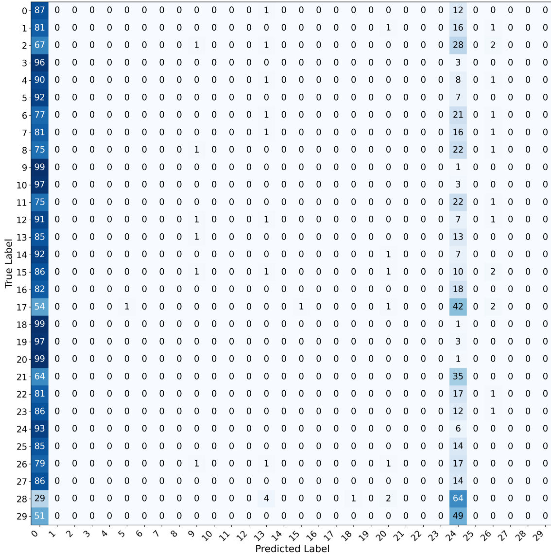
图 3-12 采用按通道 Z-score 标准化后的活动识别归一化混淆矩阵
