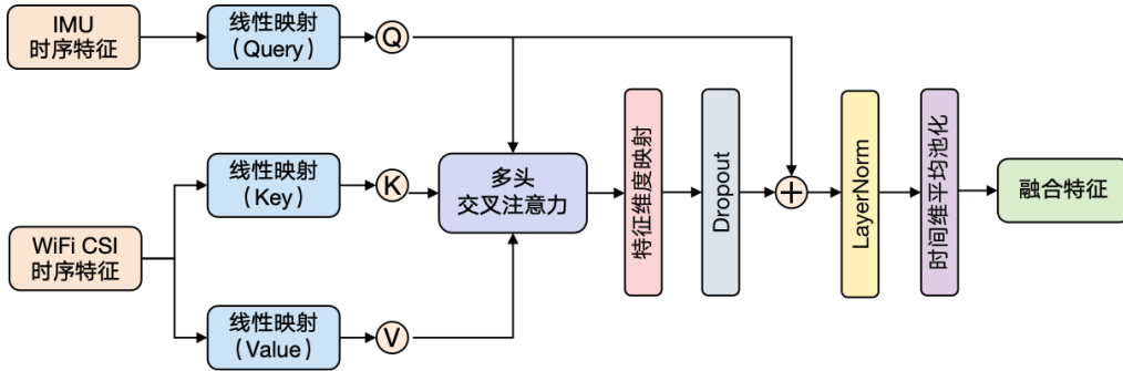
图 3-4 交叉注意力机制特征融合
