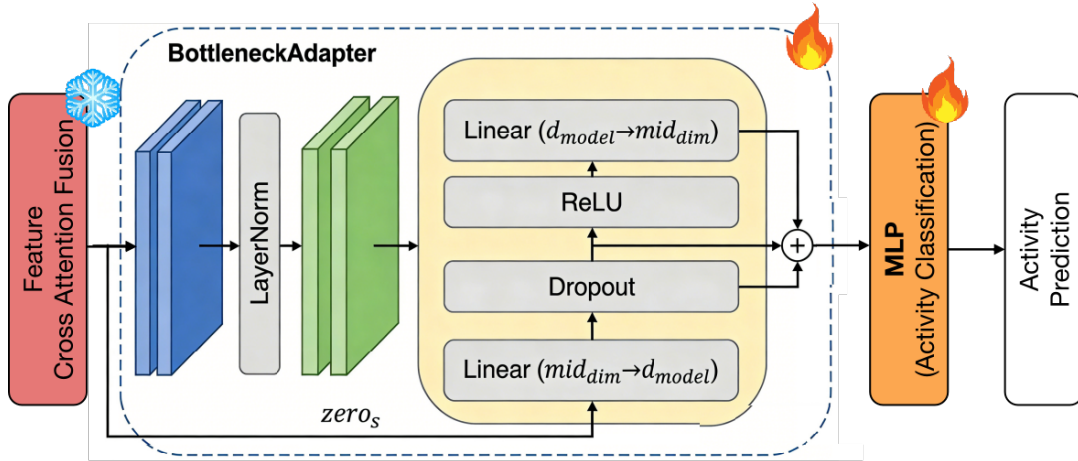
图 3-5 基于瓶颈残差结构的 Adapter 模块示意图
