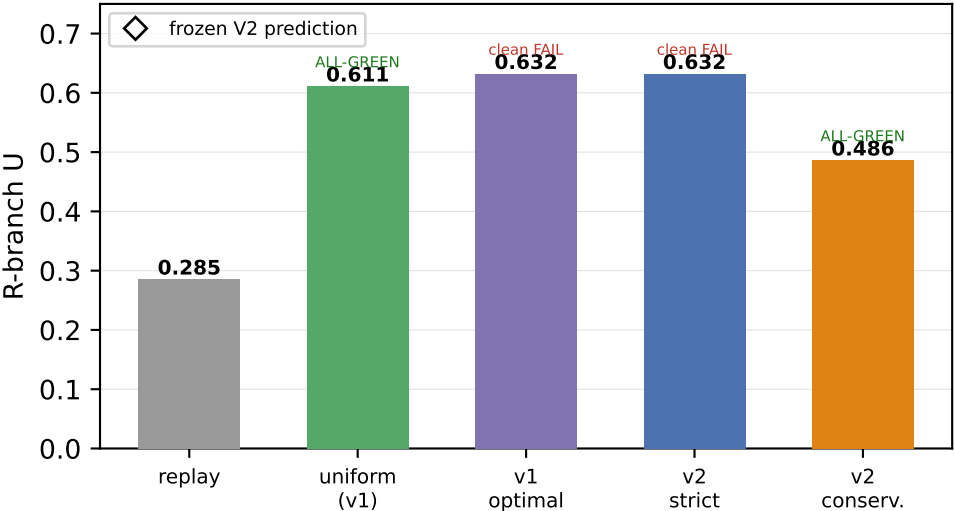
qwen3-1.7b
