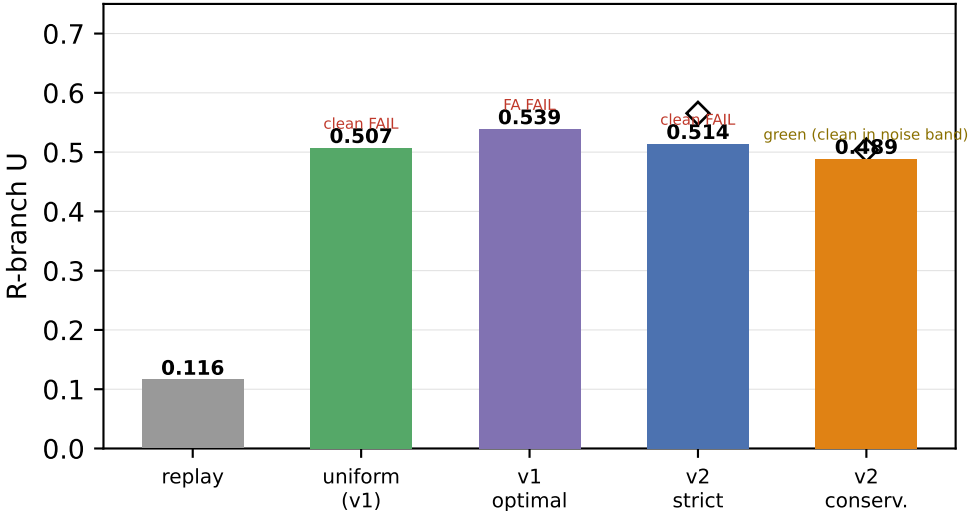
llama31-8b
