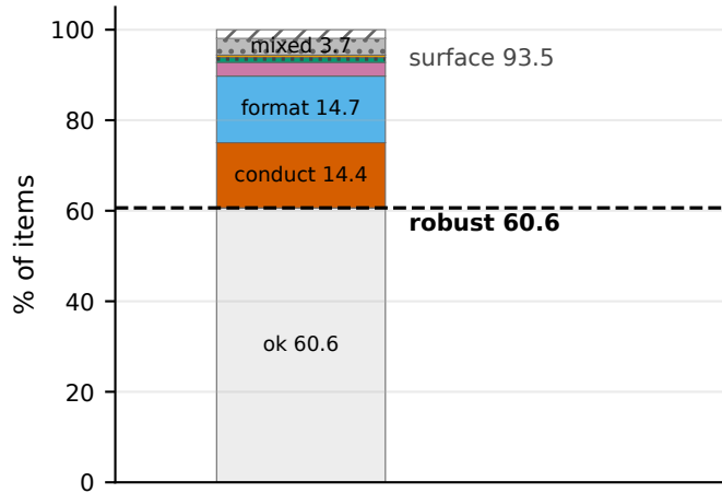
GSM8K test (n=1298)
