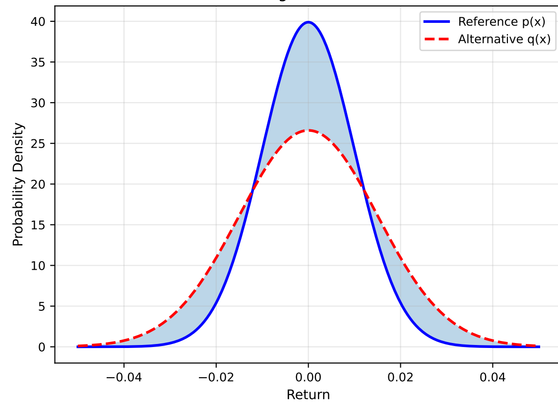
(d) Higher Uncertainty KL Divergence = 0.1277
