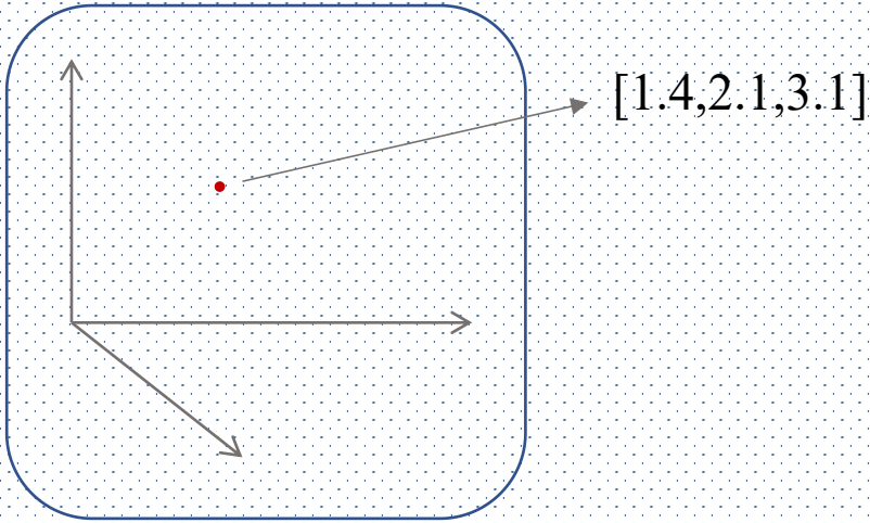
向量空间
