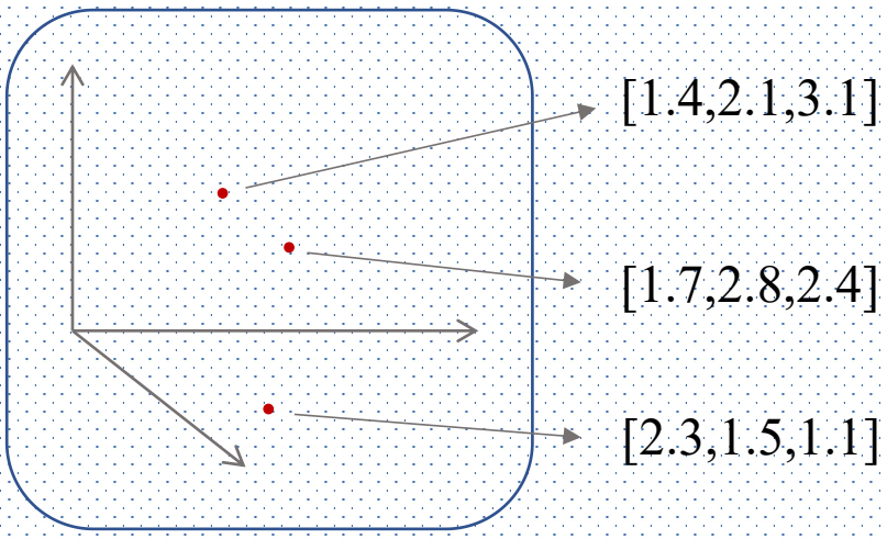
向量空间
