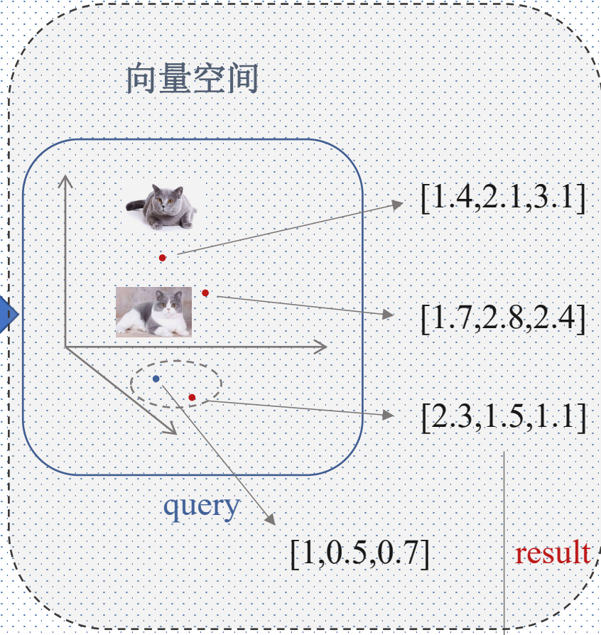
向量数据库
