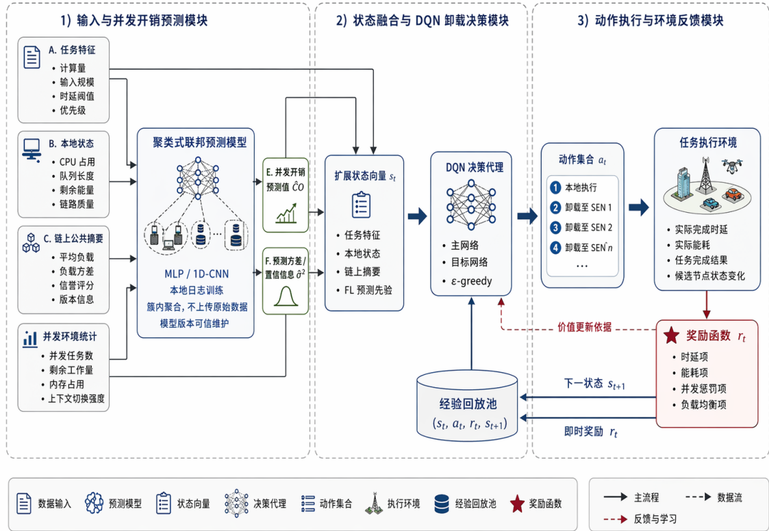
FL-DQN 预测—决策任务卸载决策算法
