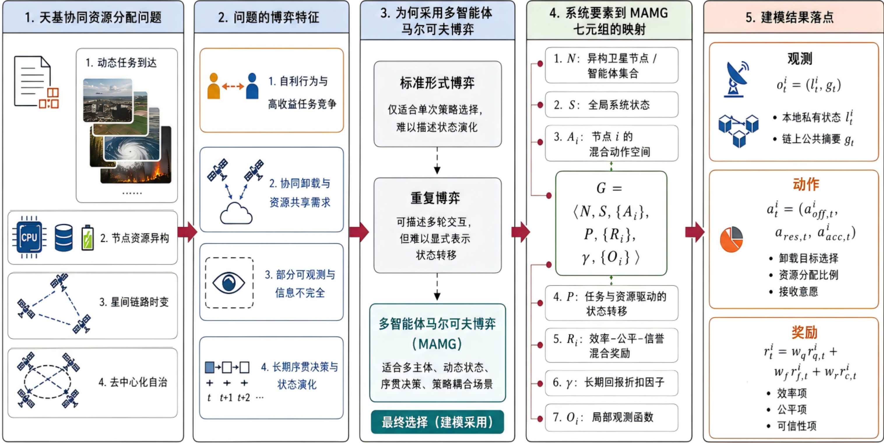
图 3-3 从系统优化问题到多智能体马尔可夫博弈的建模推导路径
