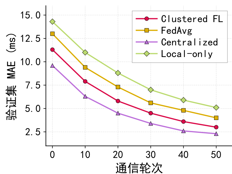
(a) 联邦训练收敛过程
