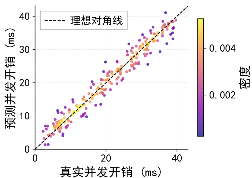
(b) 预测—真实散点密度
