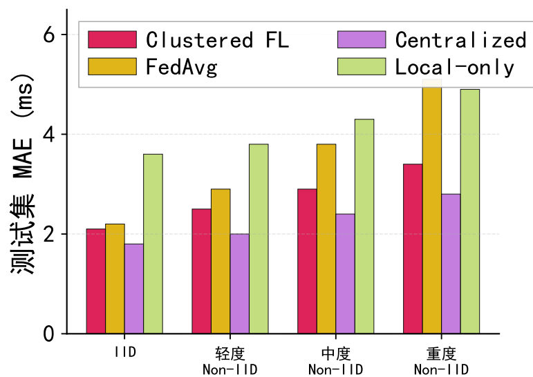
(d) 不同异构强度下的 MAE
