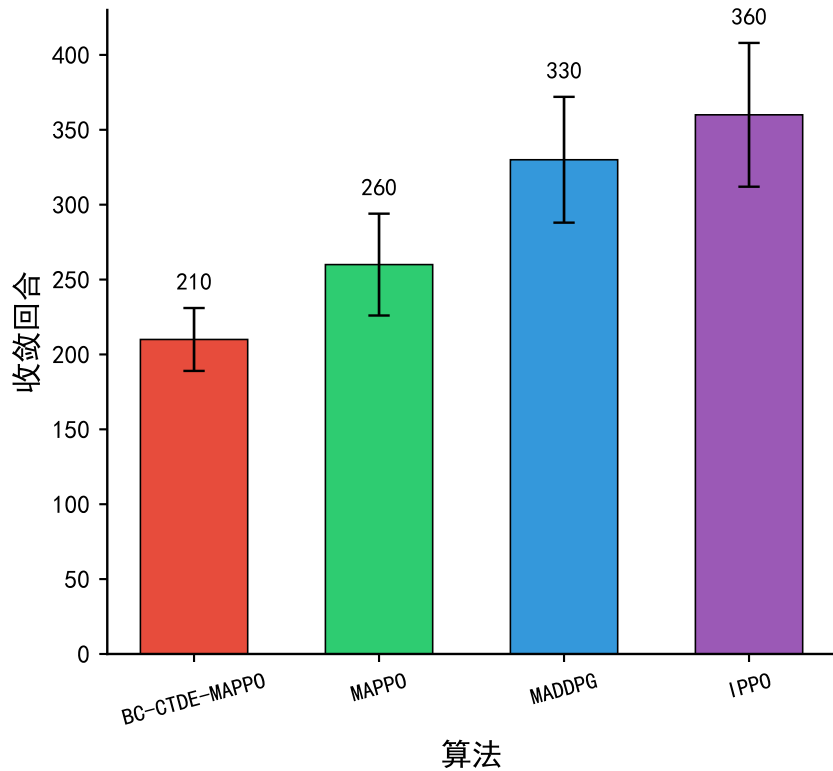
(b) 收敛回合对比
