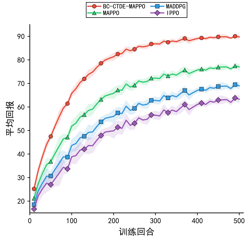
(a) 平均回报收敛曲线
